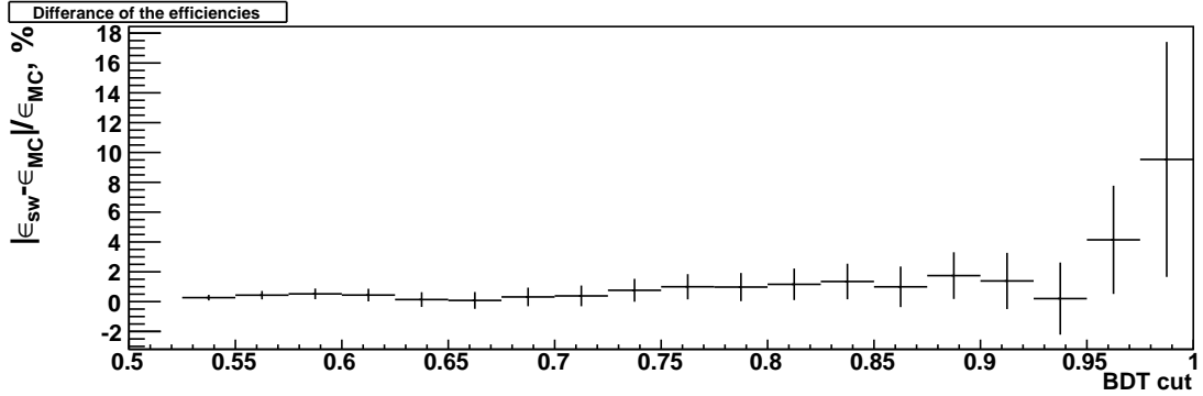
Figure 3: Différence relative de l'efficacité dans les données et le MC en fonction de la valeur de la coupure sur BDTCat . Ici, pour la désintégration D^+ \rightarrow \pi^+ \phi (\rightarrow \mu^+ \mu^-) . La coupure utilisée dans l'analyse est BDTCat \geq 0.9 .
