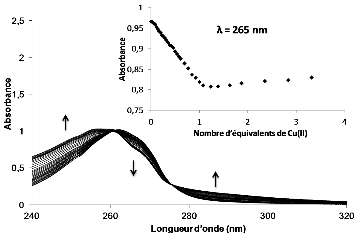
Figure 3. 19: Titrage spectrophotométrique de L^3 + Cu(ClO_4)_2 à pH 2. Solvant : H_2O ; I = 0,1 M (KCl) ; T = 25,0(2)^\circ C ; [L^3]_i = 8,94 \times 10^{-5} M ; [Cu(ClO_4)_2]_{aj.} = 8,59 \times 10^{-4} M .
