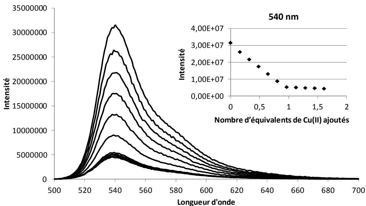
Figure 4. 18: Titrage en spectrofluorimétrie du ligand L^{14} par Cu(ClO_4)_2 . Solvant: tampon Tris pH 7,4, [L^{14}]_i = 4,63 \times 10^{-5} M , [Cu(ClO_4)_2]_{aj} = 5,05 \times 10^{-4} M , \lambda_{ex} = 522 nm .
