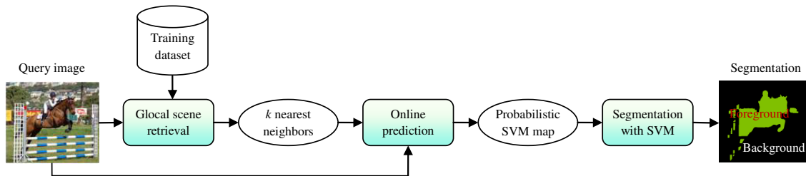
FIGURE A.4 – Schéma générique de transfert global en ligne composé de trois principaux modules algorithmiques : récupération global de scène, prédiction en ligne et segmentation avec SVM a priori.
