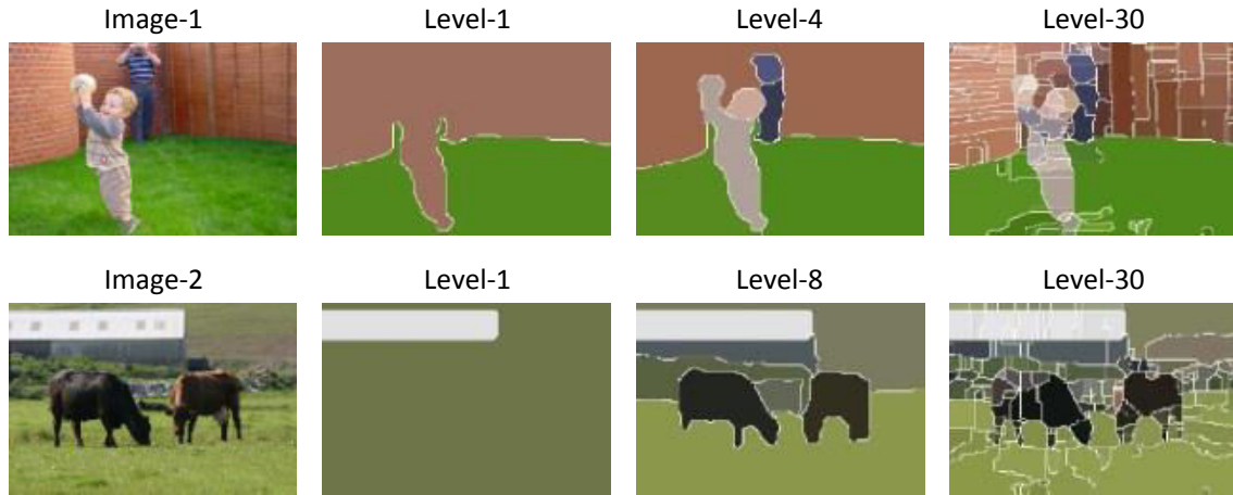
FIGURE A.6 – Deux exemples de segmentations multi-niveaux.
