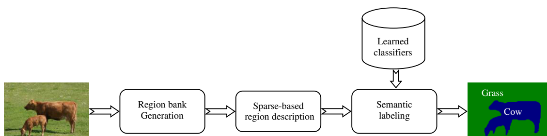
FIGURE A.5 – Schéma proposé pour la segmentation sémantique d'image.
