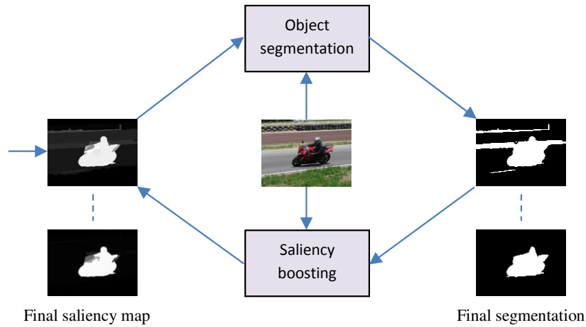
FIGURE A.3 – Schéma unifié pour obtenir conjointement segmentation d'objets et rehaussement de saillance.
