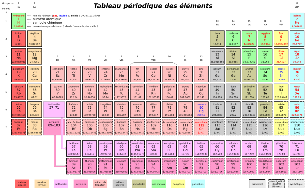
Figure 1-1 Classification périodique des éléments de Mendeleïev. Source : Wikipedia
