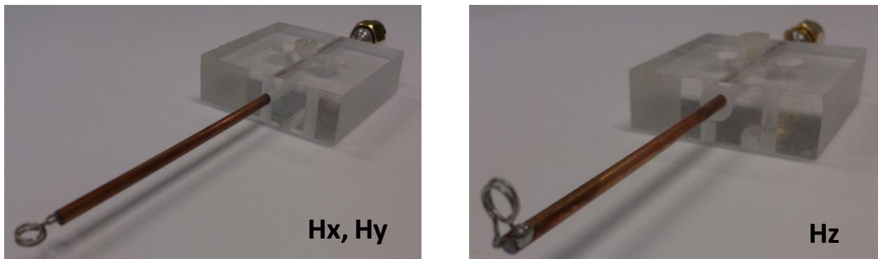
Figure IV.15 Sondes de mesure des champs magnétiques
