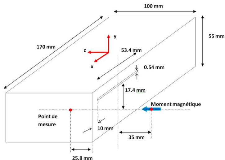
Figure III.29. Structure modélisée
