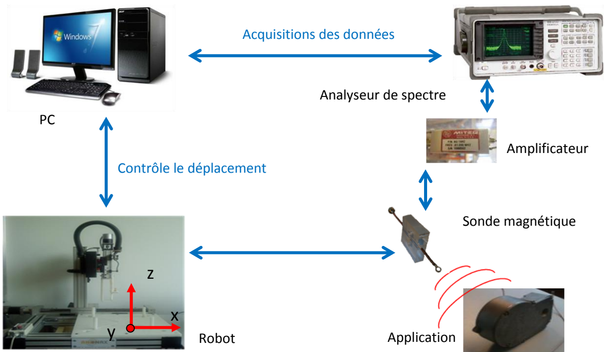
Figure IV.14 Banc champ proche développé à l'IRSEEM
