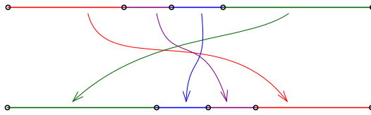
FIGURE 2.1 – Exemple d'échange d'intervalles classique
