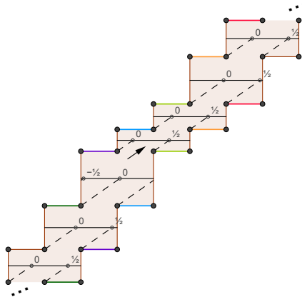
FIGURE 2.3 – L'ensemble C dans une surface en escalier.
