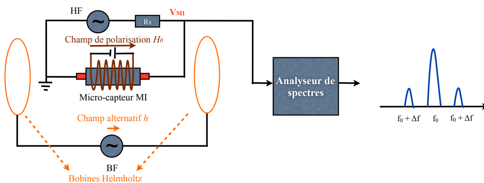
FIGURE 3-16 : Bande passante du capteur MI mesurée par un analyseur de spectre
