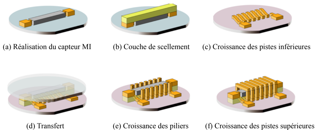
FIGURE 4-3 : Procédé de fabrication d'un micro-capteur MI avec un microsolenoides intégré
