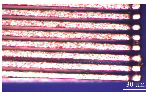
FIGURE 4-13: Micro-solenoides vu par microscope optique
