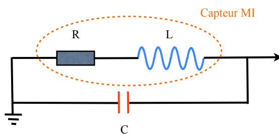
FIGURE 3-1 : Circuit résonant RLC
