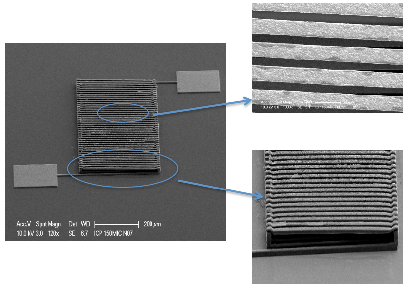
FIGURE 4-14: Micro-solenoid vue par microscope électronique à balayage
