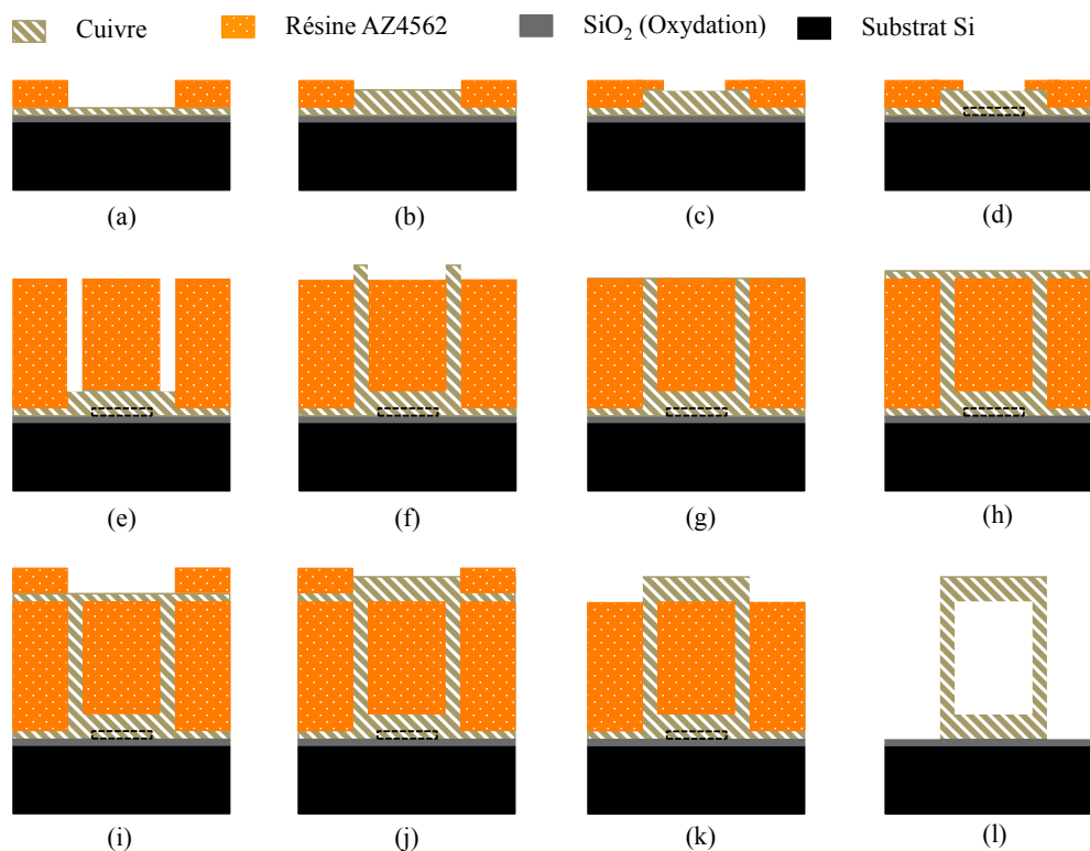
FIGURE 4-10 : Procédé de fabrication d'un microsolenoides en 3D
