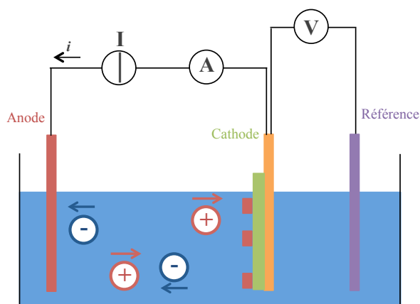
FIGURE 4-9 : Schéma de dispositif de la croissance d'électrolytique de cuivre
