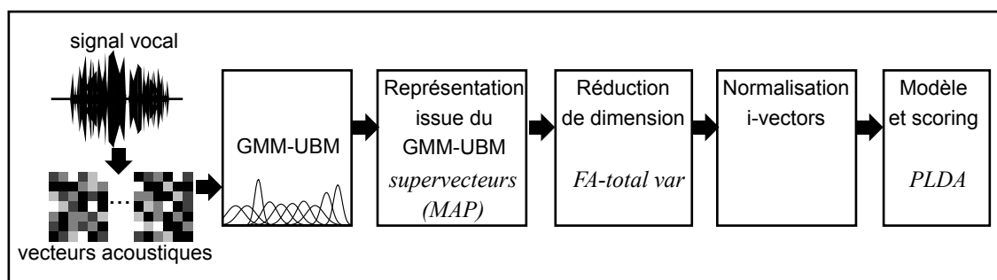
FIGURE 5.1 – Les étapes d'un système de reconnaissance du locuteur basé sur le concept de i-vectors .
