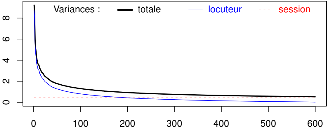
FIGURE 4.12 – Graphe spectral- \mathbf{B} du jeu de données BUT-hommes après normalisation Spherical Nuisance.
