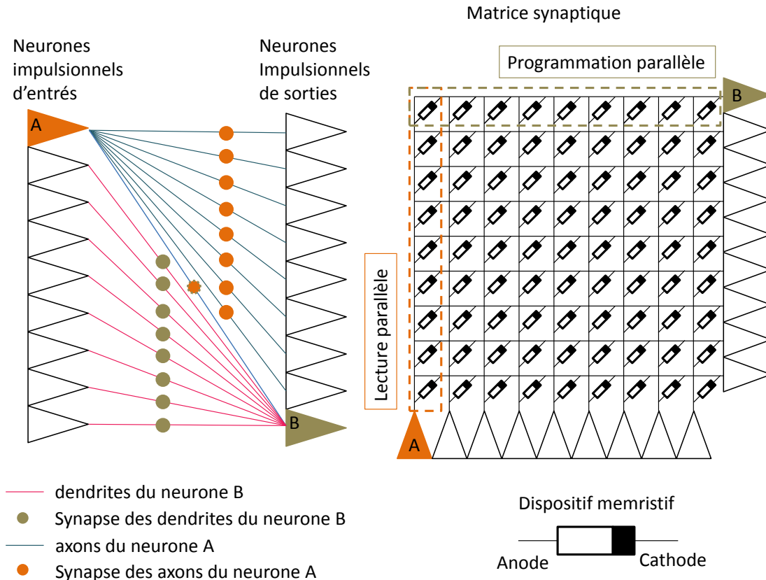
FIGURE 2 – Réseau de neurones impulsif avec 10 neurones d’entrée et 10 neurones de sortie. Grâce à la structure en crossbar, la lecture et la programmation des synapses peuvent être effectuées en parallèle.
