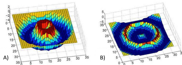
FIGURE 1.19 – Possible noyaux de la puce de convolution : Noyau de convolution permettant la détection d'un cercle ayant une circonférence A) proche de 4 pixels. B) proche de 9 pixels. (Serrano-Gotarredona et al. (2009))
