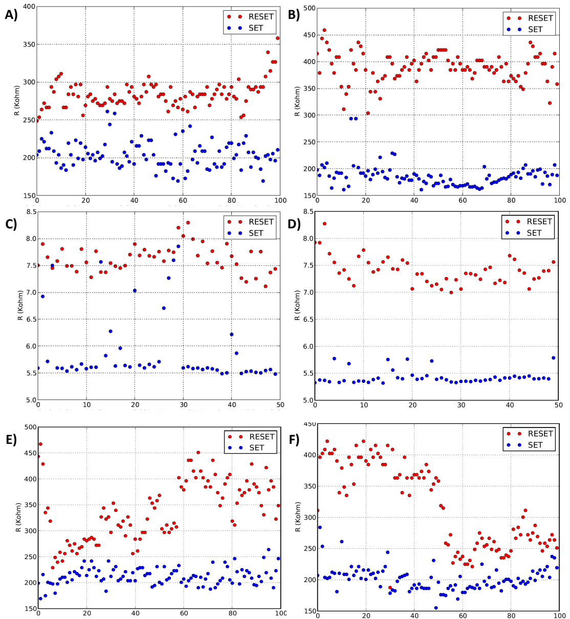
FIGURE 5.20 – Démonstration de commutations partielles sur certain dispositifs du crossbar et de la matrice. Les conditions de programmation sont présentés tableau 5.5.
