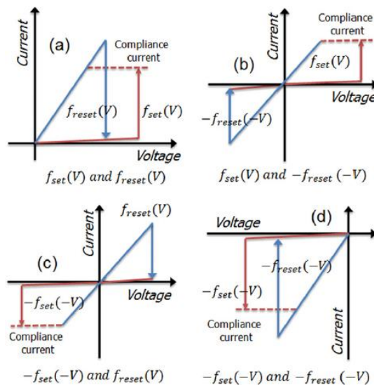
FIGURE 3.6 – Relation Tension-Courant de dispositifs bipolaires (b) et (c) et unipolaires (a) et (d) (Jeong et al. (2012))
