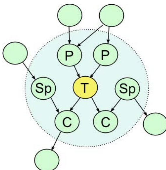
Figure 12: Exemple de couverture de Markov. L'ensemble des noeuds, liés par des arcs dirigés, correspond au réseau bayésien. La couverture de Markov de T, indiqué par un cercle pointillé, est constituée de ses parents P, ses enfants C et ses co-parents ou époux Sp.
