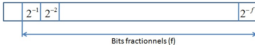
FIGURE 2.3 – Représentation d'un signal en virgule fixe avec une dynamique [-1, 1]
