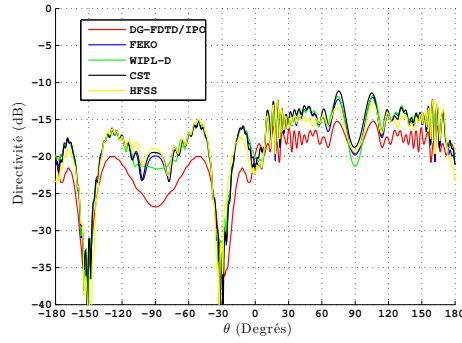
(d) CROSS-polar ( E_\phi ), plan ( y_0z ).
