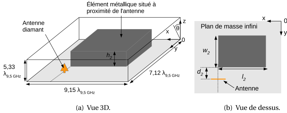
FIGURE 4.5 – Environnement proche de l'antenne diamant. l_2 = 246 \text{ mm} ; w_2 = 168 \text{ mm} ; h_2 = 144 \text{ mm} ; d_2 = 25,2 \text{ mm} .
