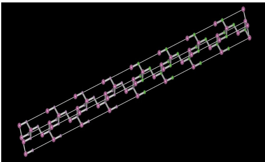
Figure 3.7. Supercellule \text{InAs}(4)\text{InP}(4) .
