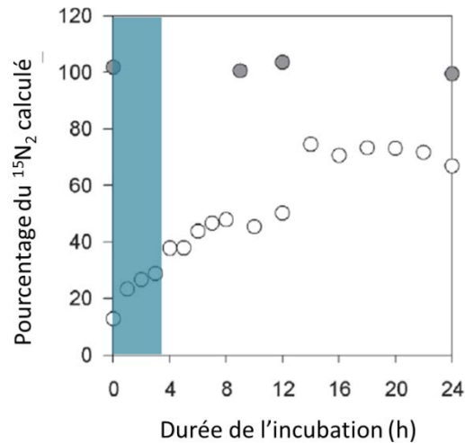
Figure 18. 15 N 2 dissous mesuré dans du YBCII après injection de 15 N 2 gazeux (point blanc) ou d'eau de mer enrichie en 15 N 2 (points gris) exprimé en pourcentage par rapport à la concentration calculée en supposant un équilibre isotopique rapide et complet. D'après Mohr et al. (2010b, Creative Commons Attribution 3.0 License). La zone bleue correspond à la durée d'incubation de nos échantillons pour la mesure des taux de fixation de N 2 .
