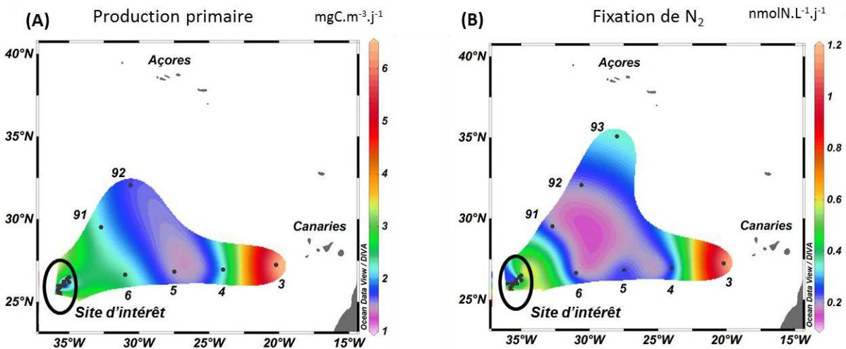
Figure 3.10. (A) Production primaire (en mgC.m -3 .j -1 ) et (B) fixation de N 2 (en nmolN.L -1 .j -1 ). Le site d'intérêt de la campagne, au centre du NASTG, est entouré en noir.
