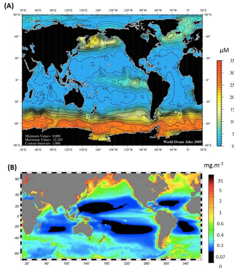
Figure 2. Moyenne annuelle des concentrations de surface (A) en \text{NO}_3^- (en \mu\text{M} ) ( World Ocean Atlas 2009, Garcia et al. 2010) et (B) en chlorophylle (en \text{mg}\cdot\text{m}^{-3} ) (National Oceanic and Atmospheric Administration, NOAA).
