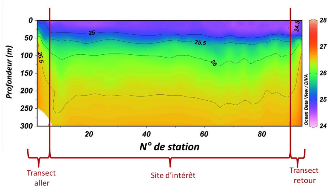
Figure 3.8. Anomalies potentielles de densité ( \text{kg}\cdot\text{m}^{-3} ) des 300 premiers mètres de la colonne d'eau en fonction des numéros des stations CTD échantillonnées durant la campagne STRASSE. Pour le site d'intérêt, cette figure représente ainsi la variabilité temporelle et non spatiale de ce paramètre.
