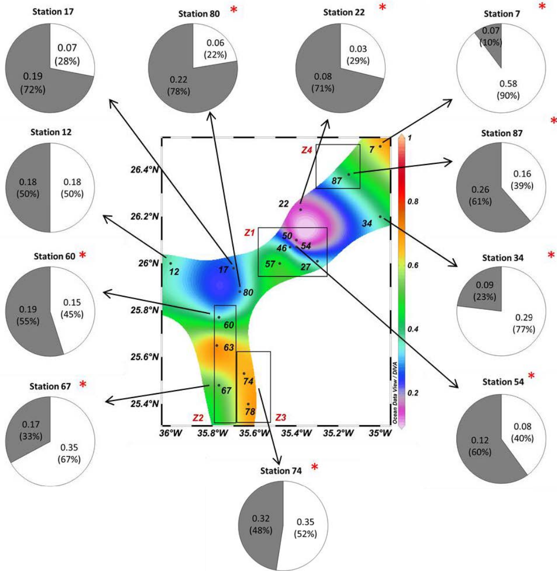
Figure 3.14. Localisation des stations du site d'intérêt avec les 4 zones (Z) encadrées sur fond de carte représentant les taux de fixation de N 2 à 10 m de profondeur. Les diagrammes secteurs représentent les taux de fixation de N 2 en période nocturne (zone grise) et diurne (zone blanche); sur les diagrammes sont indiquées les valeurs de ces taux en nmol.N -1 .j -1 ainsi que leur contribution à la fixation de N 2 journalière. Les étoiles rouges correspondent aux stations où ont été observées visuellement des colonies de Trichodesmium spp. dans les prélèvements.
