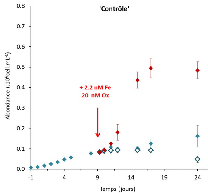
Figure 2.15. Abondance cellulaire dans le traitement 'Contrôle' transféré dans flacons de 60ml (symbole bleu ouvert), dans les bouteilles de 2L (symbole bleu plein) et après ajout de Fe en début de phase stationnaire (en rouge) (voir détails section III.8).
