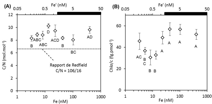
Figure 1.12. (A) Rapport molaire C/N et (B) rapport Chl a /C en \text{fg.pmol}^{-1} chez C. watsonii en phase exponentielle de croissance durant la période lumineuse en fonction des concentrations en Fe et Fe' (nM, échelle \log_{10} ). Les barres d'erreur correspondent aux écart-types associés. Des lettres différentes indiquent une différence significative des moyennes ( p < 0.05 ). La zone noire représente la région de potentielle précipitation des hydroxydes de fer.
