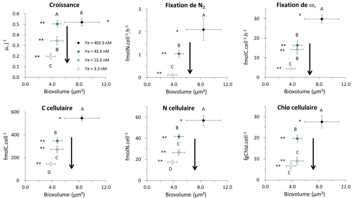
Figure 1.19. Réponse physiologique de C. watsonii en condition de limitation en fer modérée : taux de croissance ( \mu ), taux de fixation de N 2 et de CO 2 par cellule et contenus cellulaires en C, N et Chl a en fonction du biovolume. La flèche noire indique la variation observée du biovolume et des paramètres physiologiques pour une diminution de Fe de 403.3 à 43.3 nM. Un nombre différent d'étoiles indique une différence significative des moyennes du biovolume et des lettres différentes une différence significative des moyennes du paramètre considéré.
