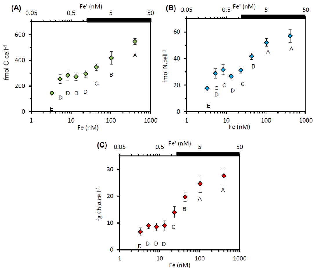
Figure 1.11. Contenus cellulaires en carbone (A) et azote (B) exprimés en fmol.cell -1 et contenus cellulaires en Chl a (C), exprimés en fg.cell -1 de C. watsonii en phase exponentielle de croissance durant la période lumineuse en fonction des concentrations en Fe et Fe' (nM, échelle log 10 ). Les barres d'erreur correspondent aux écart-types associés. Des lettres différentes indiquent une différence significative des
