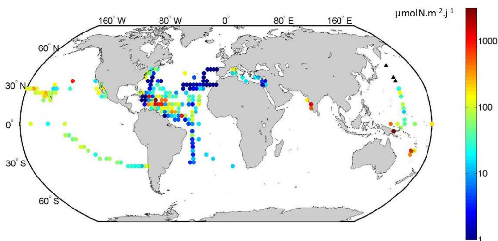
Figure 4. Moyennes géométriques des taux de fixation de N_2 intégrés sur la profondeur (en \mu\text{molN.m}^{-2}.\text{j}^{-1} selon une échelle logarithmique). Les triangles noirs correspondent à des stations explorées mais présentant des valeurs indétectables. (Luo et al. 2012, Creative Commons Attribution 3.0 License).
