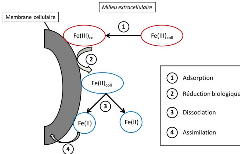
Figure 1.17. Schéma conceptuel d'un mécanisme hypothétique d'assimilation du fer(III) colloïdal (représenté par Fe(III)_{coll} ) par une cellule phytoplanctonique.
