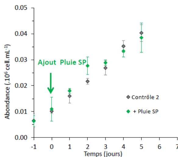
Figure 2.11. Abondances moyennes de C. watsonii dans les cultures 'Contrôle 2' (Fe = 2nM et Ox= 200 nM) et '+ Pluie SP' (ajout de pluie sans poussières).
