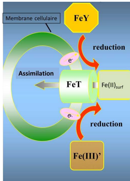
Figure 1.18. Schéma conceptuel du mécanisme de réduction du Fe(III)' et du Fe(III) complexé à un ligand (Y, tel l'EDTA) à la surface d'une cellule phytoplanctonique. Le Fe(II) libre ainsi formé à la surface des cellules ( Fe(II)_{surf} ) peut être assimilé par la cellule, via des transporteurs spécifiques ( FeT ). La diffusion possible du Fe(II) formé à la surface des cellules dans le milieu n'est pas représentée ici. D'après Shaked et al., 2005 (Copyright 2014 by the Association for the Sciences of Limnology and Oceanography, Inc.).
