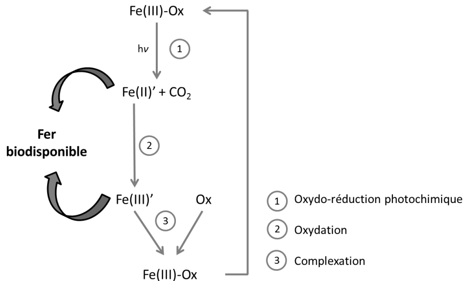
Figure 2.6. Schéma conceptuel résumant le cycle photochimique des complexes Fe(III)-oxalate (Fe(III)-Ox) dans l'eau de mer. Ox représente l'oxalate sous forme non complexé dans le milieu. D'après Sunda, comm. pers.
