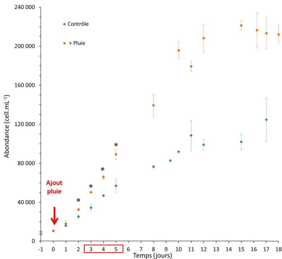
Figure 2.13. Abondances moyennes de C. watsonii cultivée en condition de limitation en fer (Fe = 2nM complexé à 200 nM d'oxalate) sans ('Contrôle') ou avec ajout d'une pluie saharienne simulée ('+ Pluie') en fonction du temps depuis l'ajout. La région encadrée correspond aux 3 jours pendant lesquels ont été effectués les prélèvements pour les mesures des paramètres permettant de caractériser la réponse physiologique de C. watsonii . Une étoile indique une abondance moyenne significativement différente dans les cultures '+ Pluie' par rapport aux cultures 'Contrôle' pour un temps donné, au cours de la phase exponentielle.
