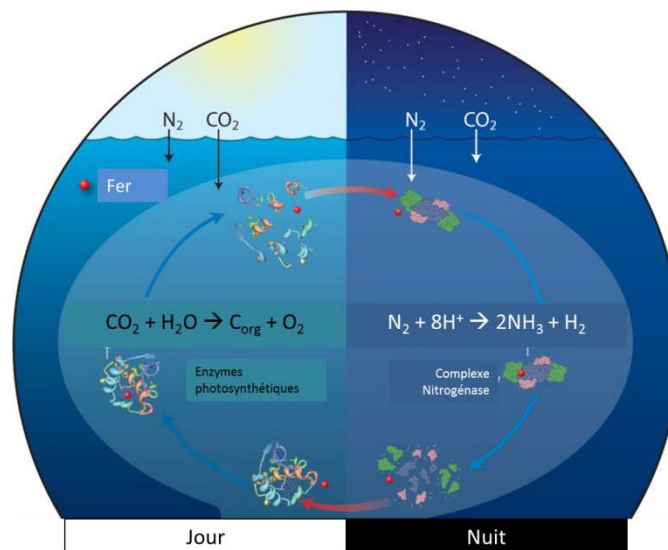
Figure 1.21. Stratégie de conservation du fer effectuée par C. watsonii . D'après M. Saito, WHOI. Les flèches rouges représente le transfert des molécules de fer libérées par les enzymes photosynthétiques et réutilisées par le complexe nitrogénase ou inversement.
