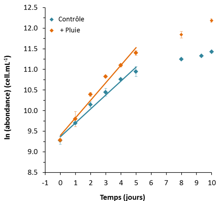
Figure 2.14. Logarithmes népériens des abondances moyennes de C. watsonii dans les cultures 'Contrôle' (2 nM de Fe et 200 nM d'oxalate) et '+ Pluie'.
