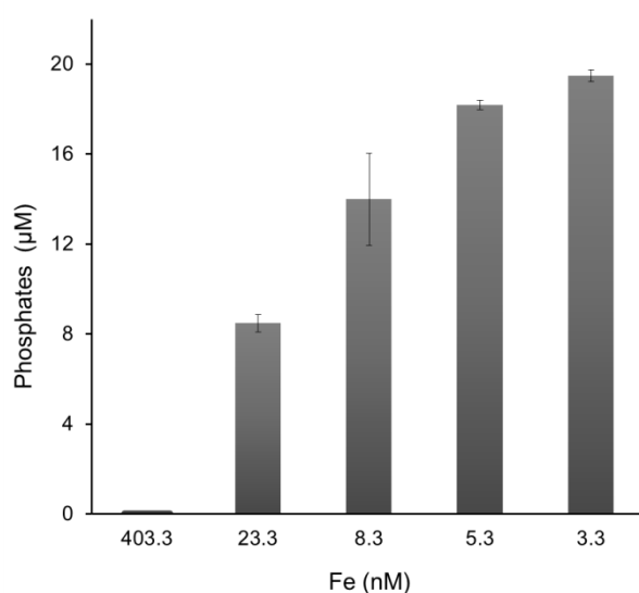
Figure 1.6. (A) Concentrations moyennes en phosphates dans les cultures en phase stationnaire, mesurées dans des cultures dont l'abondance est présentée Figure 1.5. Les barres d'erreur correspondent aux écart-types associés ( n = 3 ). La concentration initiale en phosphates était de 20 \mu\text{M} .
