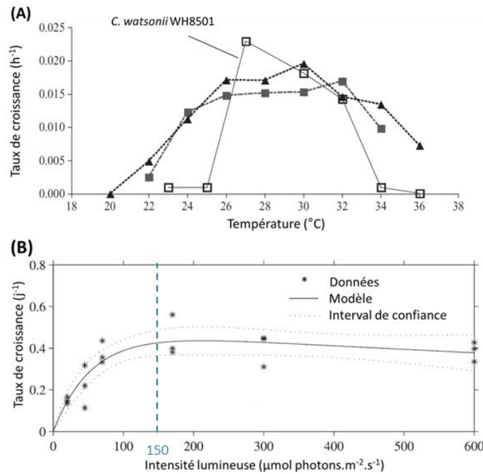
Figure 15. (A) Taux de croissance (en h -1 ) de C. watsonii WH8501 (carré blanc) en fonction de la température, d'après Webb et al. (2009) (avec la permission de John Wiley and sons, licence n° 3325410092108). (B) Taux de croissance (en j -1 ) C. watsonii WH8501 en fonction de l'intensité lumineuse d'après Goebel et al. (2008) (avec la permission de John Wiley and sons, licence n° 3403180464637).
