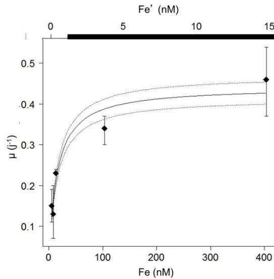
Figure 1.20. Taux de croissance moyen ( \mu , en \text{j}^{-1} ) de T. erythraeum IMS101 en fonction des concentrations en Fe et Fe' (nM) d'après Bucciarelli et al. (2013) et Rochelle-Newall et al. (2014). Les barres d'erreur représentent les écart-types associés. Le trait plein représente la régression non-linéaire de Monod (calculée à partir de Fe) et ses écart-types associés en pointillé. La zone noire représente la région de potentielle précipitation des hydroxydes de fer(III).
