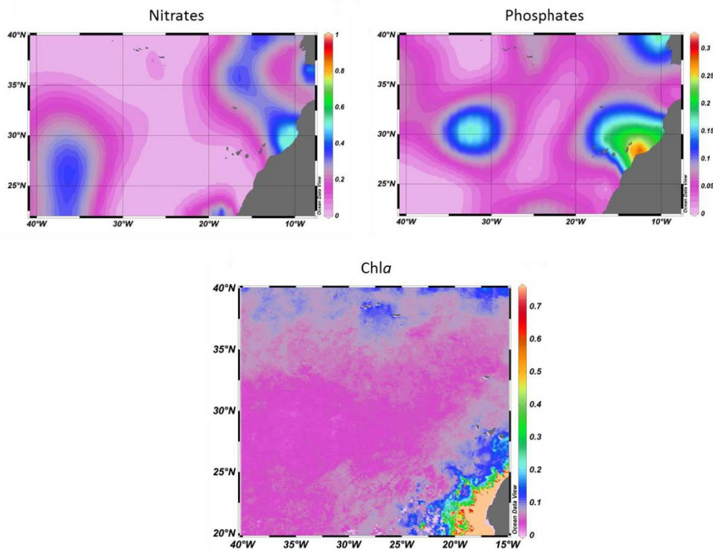
Figure 3.1. Climatologie des concentrations de surface en nitrates et phosphates pour le mois de Septembre (en \mu\text{M} , World Ocean Atlas 2009) et concentrations de surface en Chla pour le mois de Septembre 2012 (en \text{mg}\cdot\text{m}^{-3} , données du satellite MODIS).
