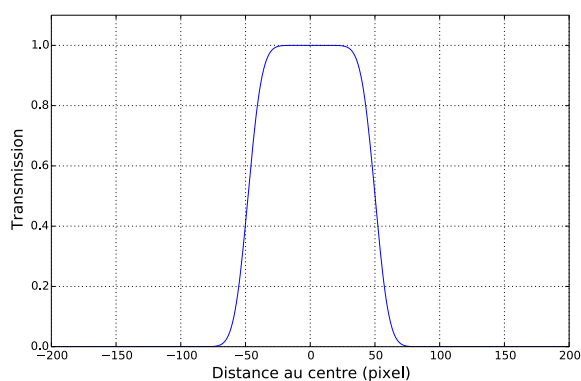
FIGURE 3.4 – Coupe du masque à bord gaussien appliqué sur les images de la FEP.
