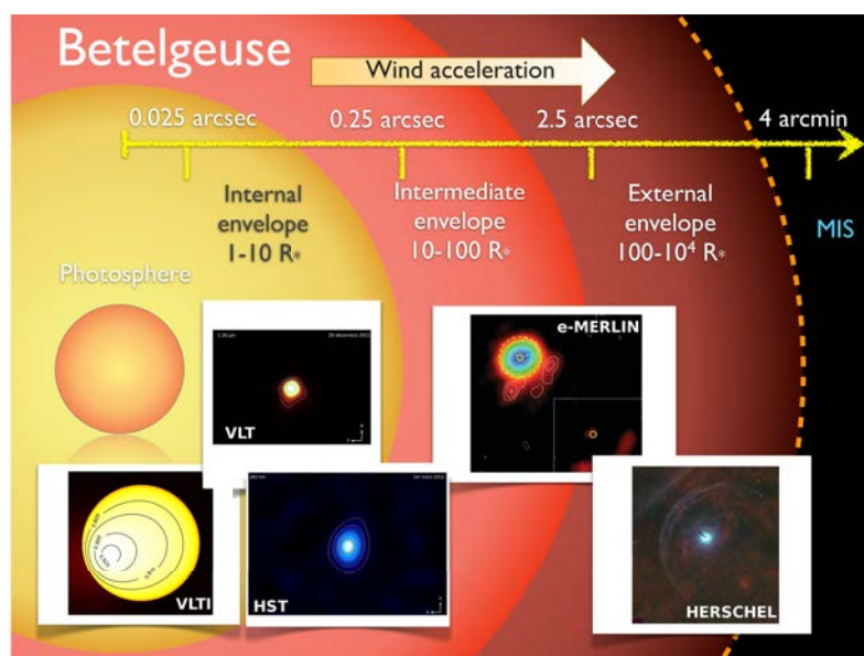
FIGURE 6.1 – Différentes couches de Bételgeuse représentées avec les images obtenues sur différents instruments. Cette figure fait écho à la Fig. 1.6 présentée dans le Chap. 1
