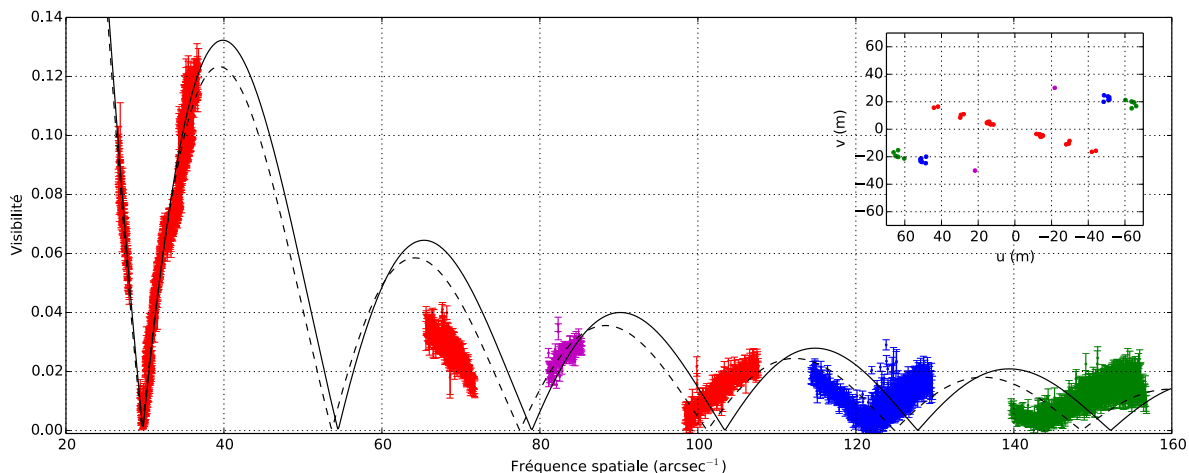
FIGURE 2.9 – Ajustement des données continuum VLTI/AMBER par des modèles analytiques simples. Insert : Couverture du plan (u, v) avec un codage couleur de l'azimut projeté. Le Nord est en haut et l'Est à gauche. Graphique principale : Les points représentent les visibilités mesurées par AMBER avec le même codage couleur que le plan (u, v) , le meilleur ajustement avec un disque UD est représenté par un trait continu et le meilleur ajustement ACB par un trait pointillés.
