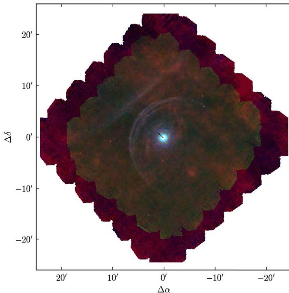
FIGURE 4.2 – Image composite trichrome des observations Herschel/PACS. Le Nord est en haut, l’Est à gauche. Le bleu correspond à l’image à 70 \mu\text{m} , le vert à 100 \mu\text{m} et le rouge à 160 \mu\text{m} . La flèche noire indique le mouvement de l’étoile à travers le MIS. (Decin et al. 2012)
