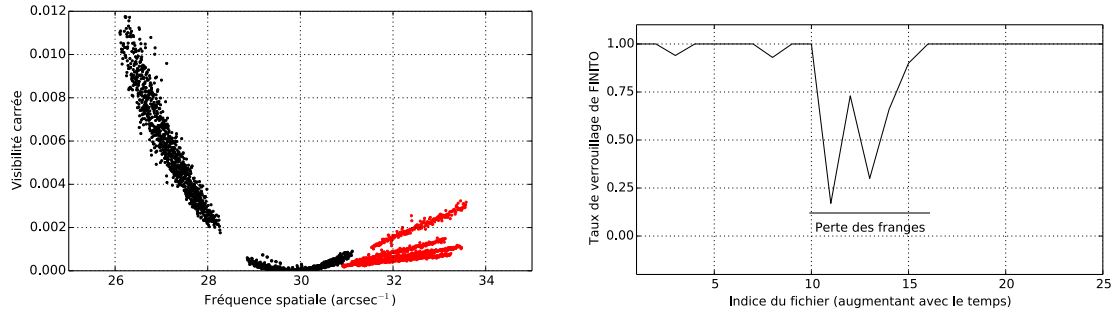
FIGURE 2.7 – Perte de verrouillage des franges par le suiveur FINITO. Gauche : Visibilités carrées de Bételgeuse mesurées par VLTI/AMBER autour du premier zéro de la fonction de visibilité. Les points noirs représentent les données non-biaisées et les rouges les données biaisées. Droite : Taux de verrouillage du suiveur de frange FINITO au cours d’une exposition. Les pertes de franges correspondent aux données représentées en rouge sur la figure de gauche.
