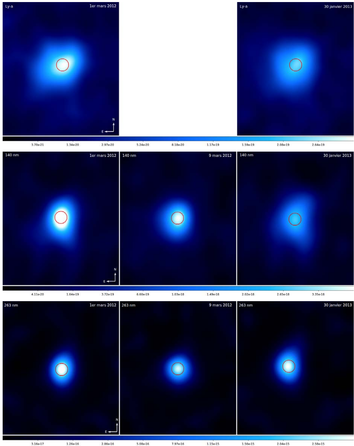
FIGURE 3.6 – Images HST/STIS réduites, déconvoluées et étalonnées. Sur chaque image le cercle rouge correspond à la photopshère infrarouge à 42 mas de diamètre et l'échelle de couleur est en racine carrée. Le filtre Ly- \alpha n'a pas été observé le 19 mars 2012
