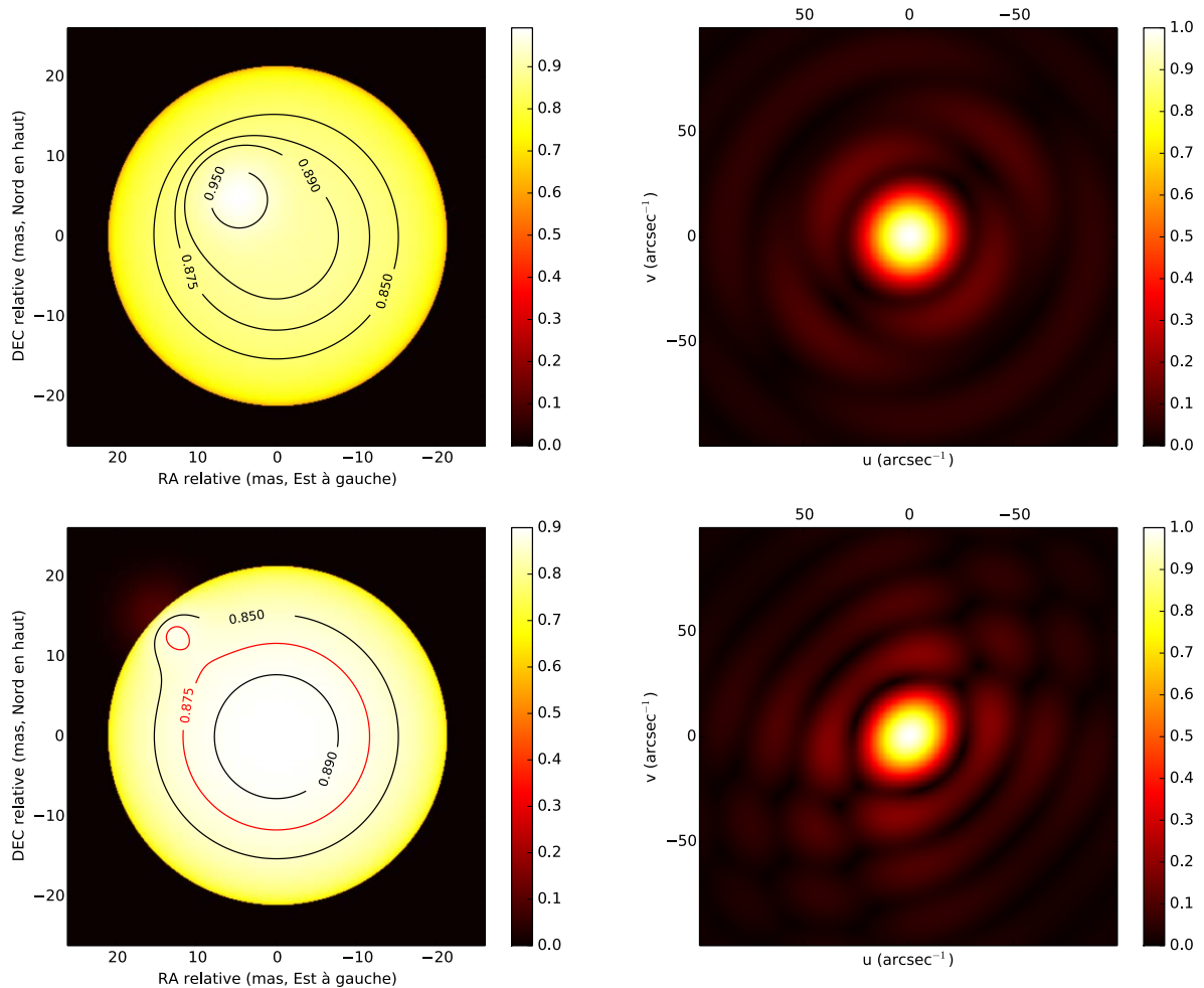
FIGURE 2.22 – Exemple de points chauds sur une étoile modélisée par un disque assombri selon une loi de puissance ( \theta_{ACB} = 42,28 \pm 0,43 ). Le point chaud est gaussien avec une FWHM à 7 mas et un flux maximal de 10% du flux maximal de l'étoile. La colonne de gauche correspond aux cartes d'intensités et celle de droite aux visibilité carrées. Haut : Point chaud à (5, 5) mas au Nord-Est. Bas : Point chaud à (15, 15) mas au Nord-Est.
