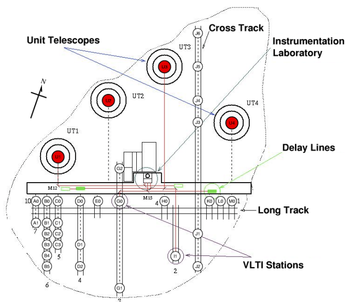
FIGURE 2.2 – Carte des différentes stations du VLTI. (Crédits : ESO)
