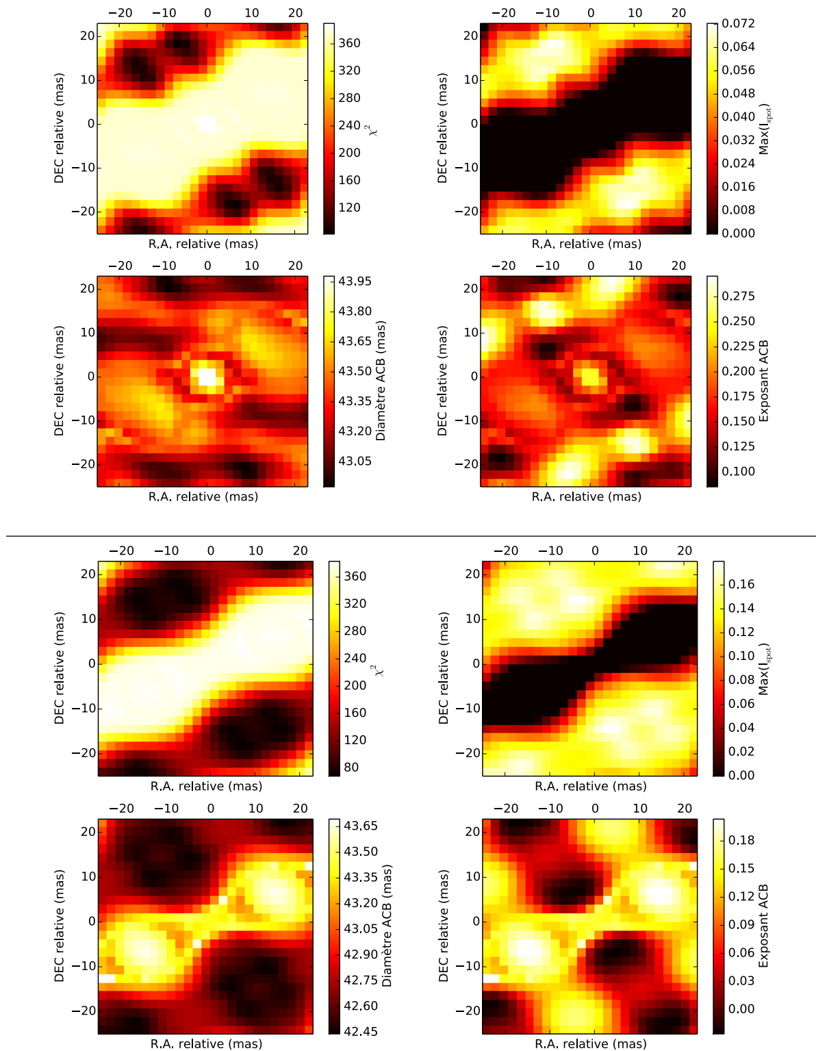
FIGURE 2.23 – Cartes exploratoires de l’ajustement des données PIONIER de janvier 2012 par un modèle de disque ACB et point chaud gaussien de FWHM 15 mas ( panneau supérieur ) et 25 mas ( panneau inférieur ). Sur chacun des deux panneaux, la première carte en haut à gauche est une carte de \chi^2 dont l’abscisse et l’ordonnée sont respectivement l’ascension droite relative et la déclinaison relative du centre du point chaud. Sur chaque cellule de la carte, trois paramètres sont ajustés. Leurs valeurs optimales sont représentées sur les trois autres cartes de chaque panneau : l’intensité maximale du point chaud en haut à droite , \theta_{ACB} en bas à gauche , et \alpha_{ACB} en bas à droite .
