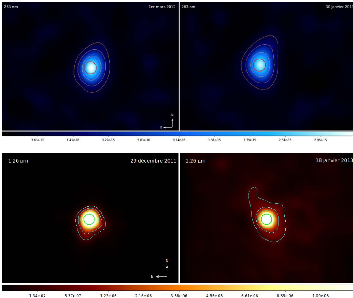
FIGURE 3.11 – Comparaison des observations HST/STIS ( haut ) et des observations VLT/NACO ( bas ). Les cercles rouges et verts correspondent à la photosphère de 42 mas de diamètre. Les contours sont décroissants d'un facteur 4 entre chaque niveau. Les contours orange d'une part et bleus d'autre part correspondent aux mêmes niveaux pour un même filtre à deux époques différentes.
