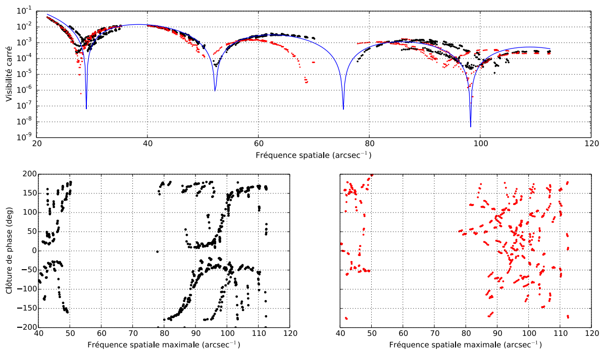
FIGURE 2.26 – Comparaison entre le meilleur ajustement de la simulation et les données PIONIER de février 2013. Haut : Visibilités. Les visibilités PIONIER sont en noir, les visibilités de la simulation RHD en rouge. Le modèle ACB correspondant au meilleur ajustement du modèle de disque ACB et point chaud gaussien (Sect. 2.3.3) est représenté par la ligne continue bleue (les visibilités du modèle avec point chaud dépendent de la direction considérée du plan (u, v) , il est donc impossible de les représenter par une ligne continue en fonction de la fréquence spatiale or la présence de ce modèle ici a pour but de guider la lecture). Bas : Les clôtures de phase PIONIER sont en noir à gauche et celles de la meilleure simulation RHD en rouge à droite.
