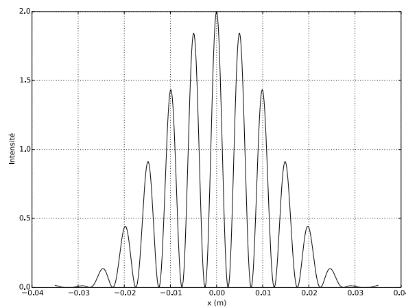
FIGURE 1.13 – Interférogramme monochromatique obtenu avec le dispositif des trous d'Young pour \lambda = 500 nm, avec des fentes d'une largeur de 5 \mu\text{m} séparées de 5 cm sur un écran situé à 1 m en prenant en compte la diffraction.
