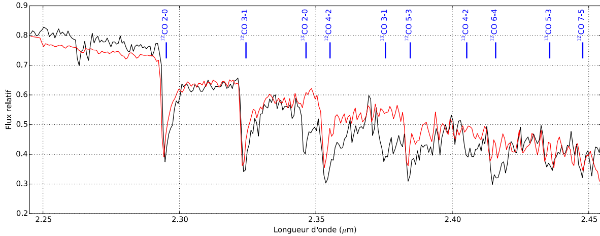
FIGURE 2.14 – Comparaison du spectre issu de l'instrument VLTI/AMBER (noir) et du modèle de MOLsphère à une couche fine (rouge). Les têtes de bande d'absorption de CO sont identifiées.
