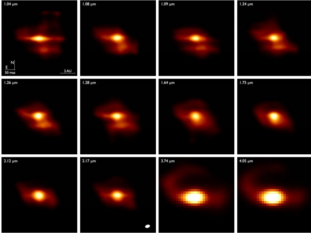
FIGURE 5.4 – Images déconvoluées de L 2 Pup par la méthode de Lucy-Richardson. L'échelle de couleur est en racine carrée. L'ellipse blanche sur l'image à 2,17 μm correspond au modèle calculé en Sect. 5.5.2.
