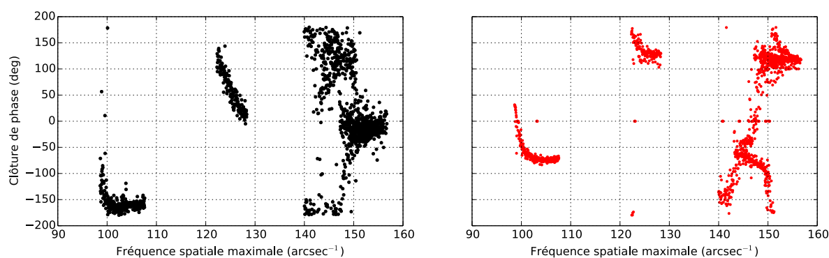
FIGURE 2.12 – Comparaison des clôtures de phase observée sur Bételgeuse par VLTI/AMBER dans le continuum (gauche) avec les clôtures de phase de la simulation RHD ajustée par les visibilités (droite).
