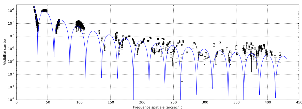
FIGURE 2.28 – Comparaison entre les données VLTI/PIONIER sur Antarès à toutes les fréquences spatiales (points noirs) et le meilleur modèle ACB déterminé par l'ajustement des fréquences spatiales < 50 \text{ arcsec}^{-1} (courbe continue bleue, voir Sect. 2.4.2).
