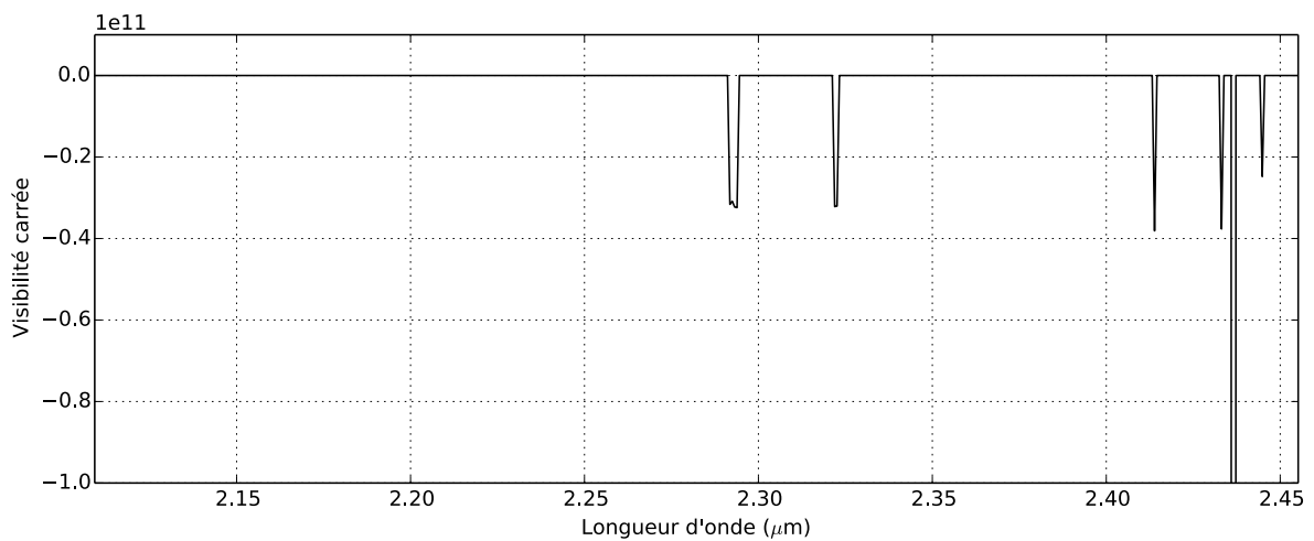
FIGURE 2.6 – Exemple de visibilités carrées représentées en fonction de la longueur d'onde. Pour certains canaux spectraux, des valeurs de l'ordre de -10^{11} sont obtenues et doivent être ignorées.
