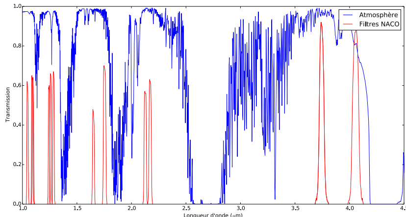
FIGURE 5.5 – Transmissions des 12 filtres à bande étroite de l'instrument NACO et de l'atmosphère terrestre (Lord 1992)
