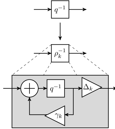
FIGURE 1.7 – La \rho DFIIt par d'une DFIIt et change tous les q^{-1} en \rho_k^{-1} .
