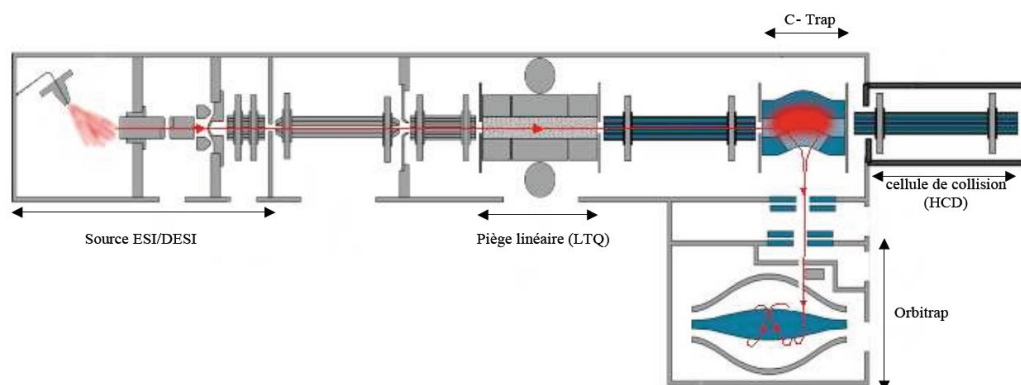
Figure 9. Schéma du LTQ-Orbitrap XL TM de ThermoFisher avec le trajet des ions
