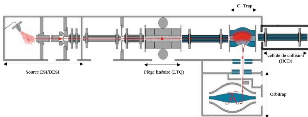
Figure 9. Schéma du LTQ-Orbitrap XL TM de ThermoFisher avec le trajet des ions
