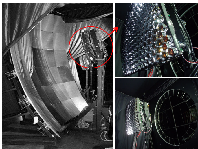
FIG. 1.28 – Photographie d'un télescope à fluorescence, le miroir sphérique de 3,5 m × 3,5 m est visible à gauche, le réseau de photomultiplicateurs (22 lignes × 20 colonnes) constituant le plan focal est présenté en haut à droite et la lentille de collimation, ainsi que le filtre UV permettant de protéger le télescope sont visibles en bas à droite.
