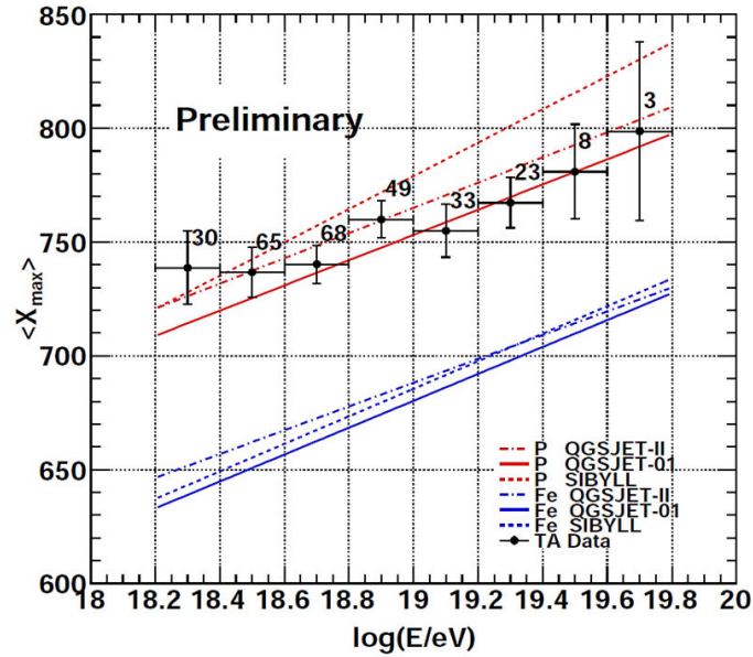
FIG. 1.11 – X_{\max} mesurés par TA en fonction de l'énergie. Les lignes indiquent les résultats de simulations pour le fer (en bleu) et le proton (en rouge) effectuées avec différents modèles hadroniques. La composition est compatible avec des protons à haute-énergie. La figure est extraite de [21].
