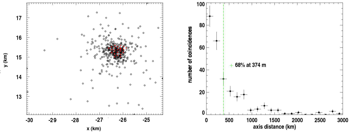
FIG. 4.15 – À gauche : positions des cœurs particules des 329 coïncidences données par le SD, indiquées par les losanges noirs, les stations radio d'AERA-I sont indiquées par les croix rouges. À droite : distribution des distances moyennes entre le barycentre des stations AERA sélectionnées pour un évènement donné et l'axe de la gerbe pour les 329 coïncidences.
