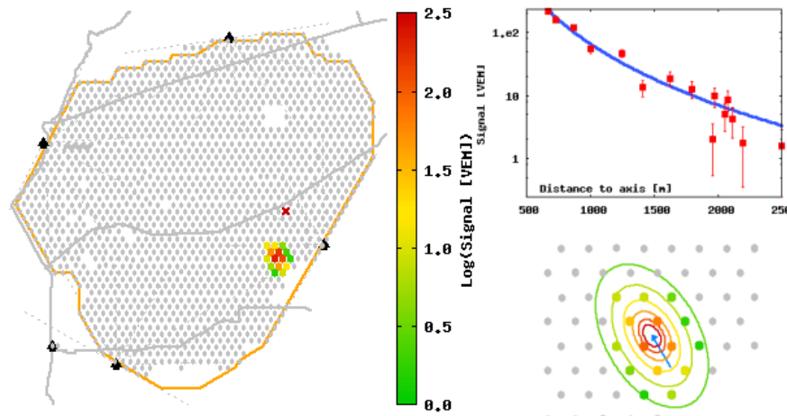
FIG. 1.26 – Évènement choisi arbitrairement détecté par le réseau de surface. À gauche : empreinte au sol de la gerbe superposée à la carte de l'observatoire, en haut à droite : distribution latérale ajustée par une fonction NKG, en bas à droite : zoom sur l'empreinte de la gerbe au sol. L'échelle colorée représente l'intensité du signal mesuré par les cuves Cherenkov en VEM (Vertical Equivalent Muon), correspondant à la lumière déposée par un muon vertical traversant la cuve.
