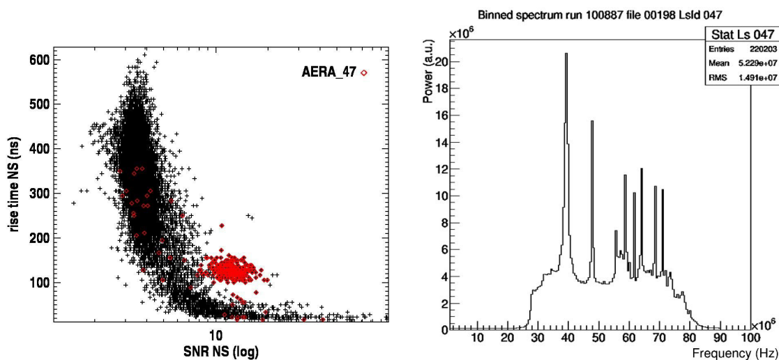
FIG. 4.36 – À gauche : comparaison du temps de montée des 185 coïncidences avec leur SNR (en log) pour la polarisation NS, les valeurs correspondant à la station AERA_47 sont indiquées en rouge. La population secondaire observée est peuplée par les contributions de cette station. À droite : spectre moyenné sur toutes les traces du fichier de données 198 du run 100887 détectées par la station AERA_47, de nombreuses contributions de forte intensité sont visibles.
