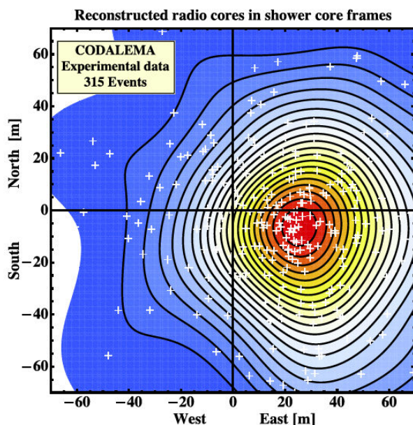
FIG. 1.22 – Positions relatives des cœurs radio par rapport aux cœurs particule pour 315 gerbes CODALEMA (croix blanches). Chaque cœur particule est centré en (0,0) . Le code couleur représente la densité de cœurs radio à un endroit donné de la carte. On observe un décalage systématique du cœur radio vers l'est. La figure est extraite de [43].
