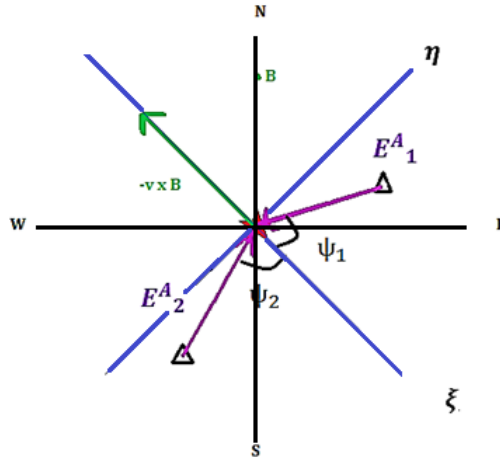
FIG. 2.28 – Représentation du champ électrique induit par l'excès de charge, \vec{E}_A^A en violet, pour deux stations représentées dans le repère défini dans la figure 2.27. Les directions projetées dans le plan du sol du champ électrique dû à l'excès de charge pour chaque position d'antenne sont définies par les angles \Psi_1 et \Psi_2 .
