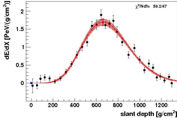
FIG. 5.12 – Profil longitudinal de l'évènement Coihueco 1018 du run 5262 : perte d'énergie en fonction de l'épaisseur d'atmosphère traversée. L'ajustement du profil par la fonction de Gaisser-Hillas est indiqué en rouge.
