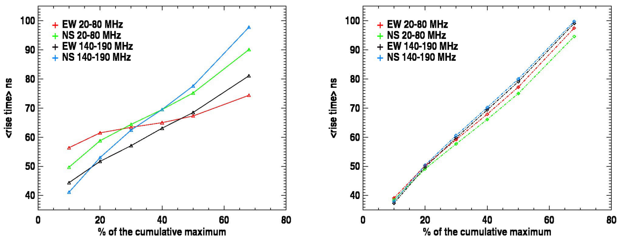
FIG. 3.8 – À gauche : moyennes des temps de montée de l'échantillon gerbe en fonction du pourcentage de maximum de la cumulative, C_{\max} , allant de 10 % à 70 % utilisé en borne supérieure du calcul du temps de montée, la borne inférieure étant fixée à C_{\min} = 0 . pour quatre lots de traces : EO filtrées dans la bande 20-80 MHz (en rouge) et 140-190 MHz (en noir), NS filtrées dans la bande 20-80 MHz (en vert) et 140-190 MHz (en bleu). À droite, idem pour l'échantillon bruit de fond en pointillé.
