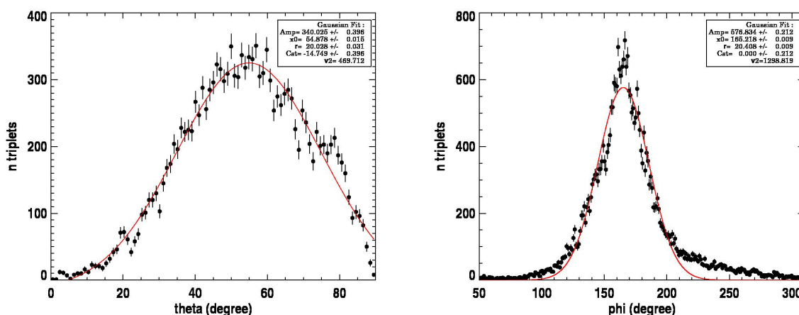
FIG. 4.26 – Exemple de distributions angulaires obtenues pour un évènement, à gauche pour \theta et à droite pour \phi . Les ajustements gaussiens donnent pour cette exemple une direction d'arrivée de (\theta; \phi) = (54, 9 \pm 20; 166, 9 \pm 20)^\circ . Les dispersions des distributions sont dues au fait que toutes les traces de l'évènement sont utilisées pour la reconstruction par triplets, sans sélection préalable, même celles correspondant à du bruit, ceci afin de réduire la probabilité de reconstruire un évènement bruit dans la même direction que celle de l'évènement SD étudié.
