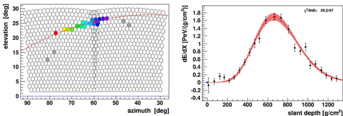
FIG. 1.29 – Évènement choisi arbitrairement, détecté par deux miroirs de Coihueco. À gauche : trace de lumière de fluorescence détectée par le réseau de PMs en fonction de l'azimut et de l'élévation, l'échelle de couleur représente le temps relatif de détection de la trace ; à droite profil longitudinal, perte d'énergie en fonction de la profondeur d'atmosphère, ajusté par la fonction de Gaisser-Hillas.
