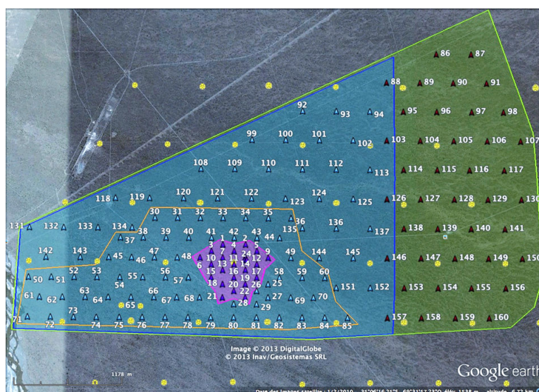
FIG. 2.12 – Carte d’AERA au cours de l’année 2014. AERA-I, installé en 2010 et composé de 24 stations espacées de 144 m, est présenté dans la zone violette; AERA-II, installé en 2013 et composé de 100 stations espacées de 250 m pour les stations incluses dans la ligne orange et 375 m pour les autres, est présenté dans la zone bleue. La future phase 3 d’AERA, prévue fin 2014/début 2015, est indiquée par la zone vert. Les cuves Cherenkov de l’Infill sont indiquées en jaune.
