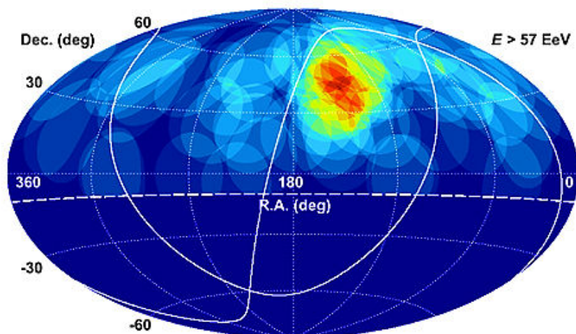
FIG. 1.7 – Directions d’arrivée des évènements d’énergie supérieure à 57 EeV détectés par TA. L’échelle de couleur indique le nombre d’évènements reconstruits dans un cercle de 20^\circ . La figure est extraite de [19].
