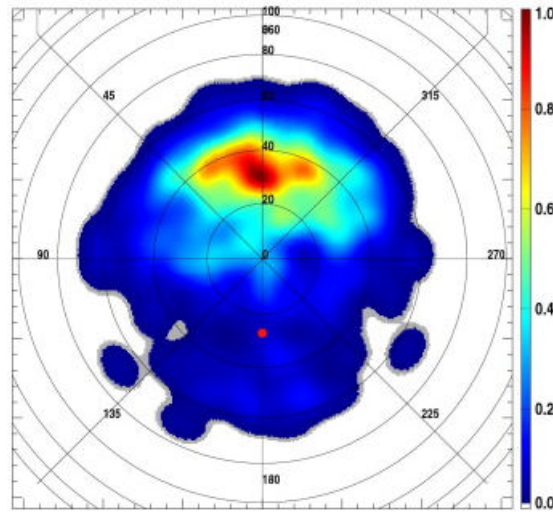
FIG. 1.18 – Distribution des directions d'arrivée d'évènements vus par CODALEMA. Comme attendu du comportement de l'effet géomagnétique, un excès d'évènements est observé en provenance du nord, dans la direction opposée à celle du champ géomagnétique à Nançay, indiqué par le point rouge. La figure est extraite de [42].
