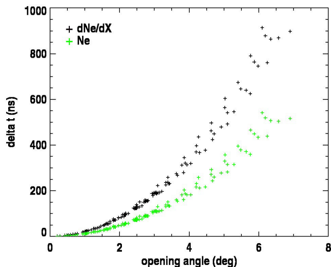
FIG. 5.6 – Comparaison des durées \delta t_j des signaux issus de N_e en vert e tdN_e/dX en noir vus par un observateur au sol, émis sur les points M_i en fonction de l'angle d'ouverture des stations. La durée des signaux est définie par la durée séparant les deux points du signal correspondant à la largeur à mi-hauteur.
