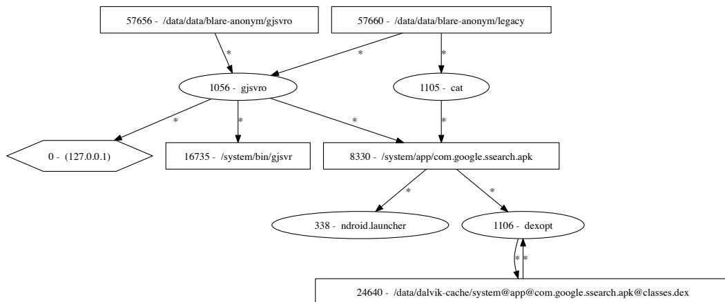
FIGURE 5.2 – S1 : sous-graphe en commun des échantillons de DroidKungFu 1
