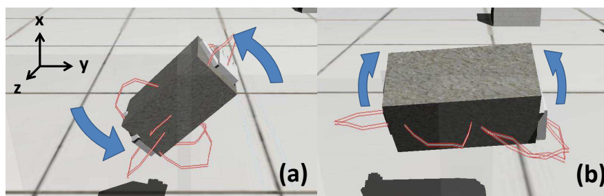
Figure A.3 – Rotation d'un objet virtuel avec l'approche basée contrainte de la prise magnétique . (a) Rotation autour de l'axe de profondeur en utilisant la position relative entre les deux mains. (b) Rotation autour de l'axe de saisie en utilisant le moment de l'interface de droite.
