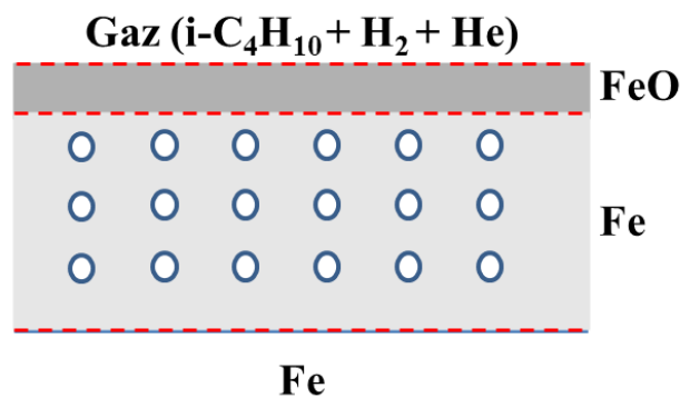
Figure III.61 : Réduction des oxydes de fer sous ( i\text{-C}_4\text{H}_{10} + \text{H}_2 ) et création de pores
