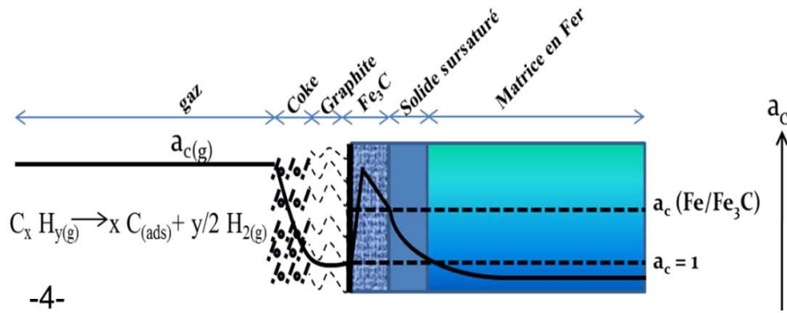
Figure III.3 : Mécanisme de formation des particules catalytiques sur le fer et les aciers faiblement alliés [88]
