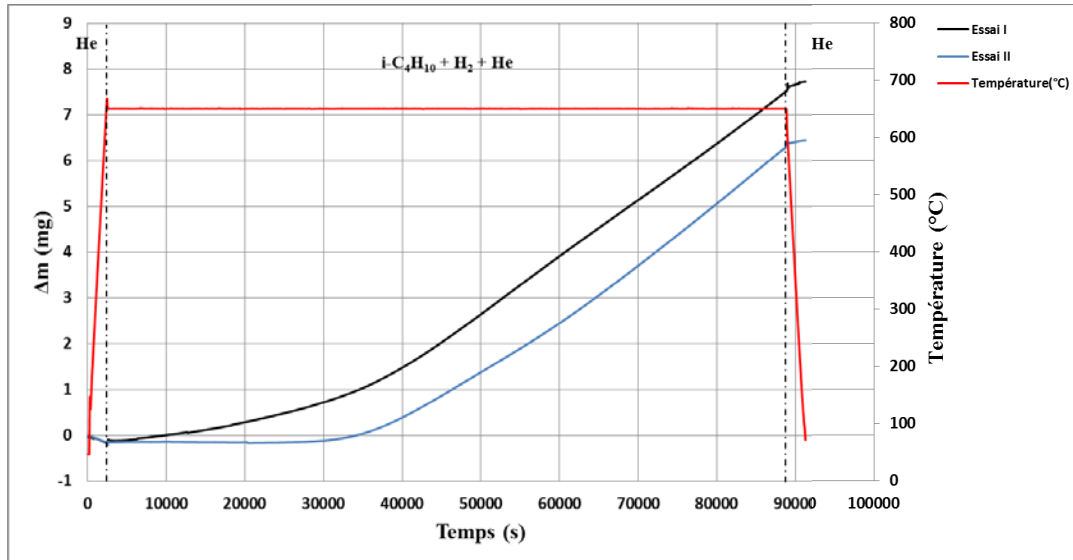
Figure III.18 : Variation de masse d'un échantillon de fer, test de corrosion sous ( i\text{-C}_4\text{H}_{10} + \text{H}_2 + \text{He} ) à 650 °C
