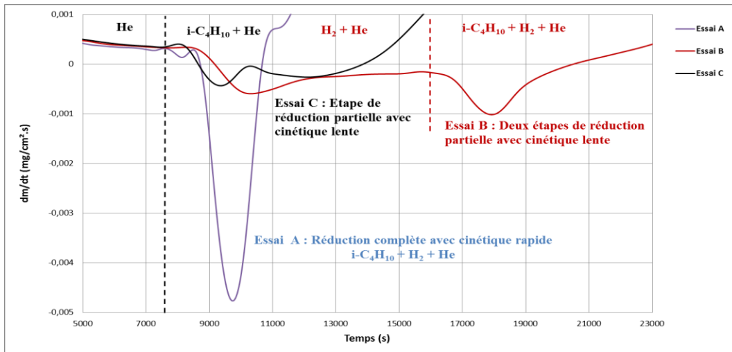
Figure E.2 : Courbes cinétiques de différents essais réalisés avec des mélanges gazeux différents
