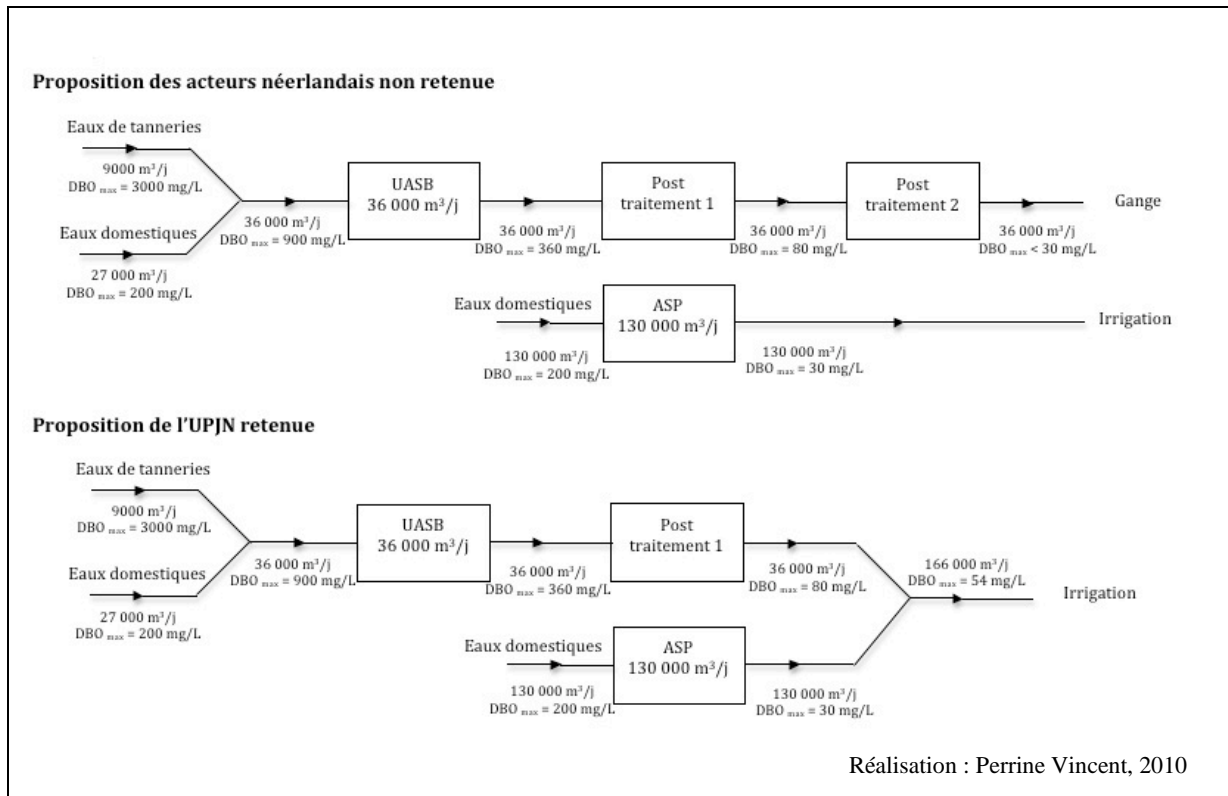
Schéma 6 – raisonnement menant au choix de post traitement et de la destination des eaux traitées
