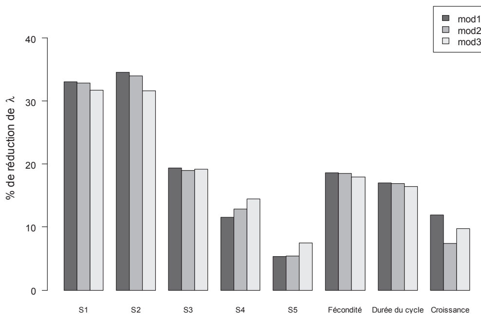
Figure IV-10 : Sensibilité du taux d'accroissement asymptotique annuel \lambda de la population de G. fossarum aux paramètres de survie, de fécondité et de croissance (réduction de 10 %).
