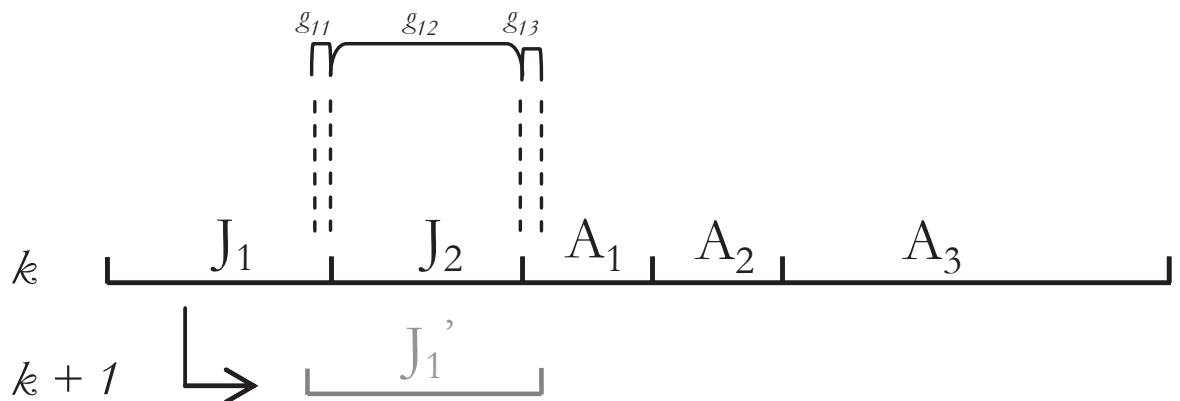
Figure IV-7 : Illustration théorique du calcul des taux de transition pour la classe J1.
