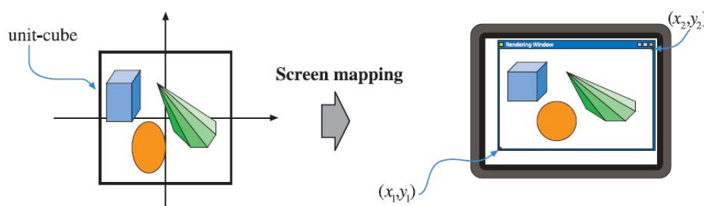
Figure 3.9 – Projection de la scène sur une fenêtre de l'écran.
