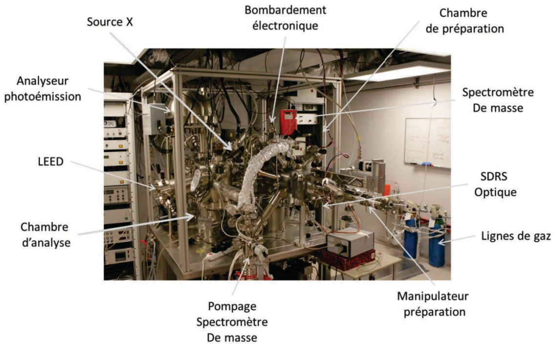
Figure 2.1. Photographie du bâti ultra-vide utilisé. Les éléments essentiels utilisés lors de ce travail sont marqués d'une flèche.
