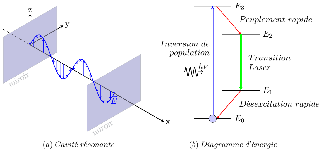
FIGURE I)-19 – (a) : Phénomène de réflexion du champ électrique \vec{E} entre deux miroirs. (b) : Inversion de population par pompage dans un système atomique à quatre niveaux conduisant à une émission laser.
