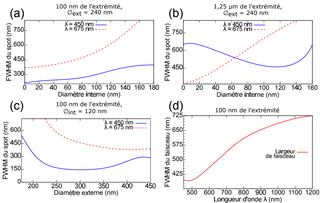
FIGURE II)-12 – Evolution de la largeur à mi-hauteur (FWHM) du faisceau, pour un indice de réfraction fixé à n = 1,56 , aux longueurs d'onde \lambda = 450 nm et \lambda = 675 nm dans les cas de nanotube au diamètre externe fixé à 240 nm en fonction du diamètre interne à (a) : 100 nm et (b) : 1,25 \mu\text{m} . (c) : Pour un nanotube au diamètre interne fixé à 120 nm, évolution de la largeur de faisceau en fonction du diamètre externe. (d) : Largeur de faisceau pour un nanotube de diamètres externe et interne respectivement de 240 nm et 120 nm en fonction de la longueur d'onde de propagation.
