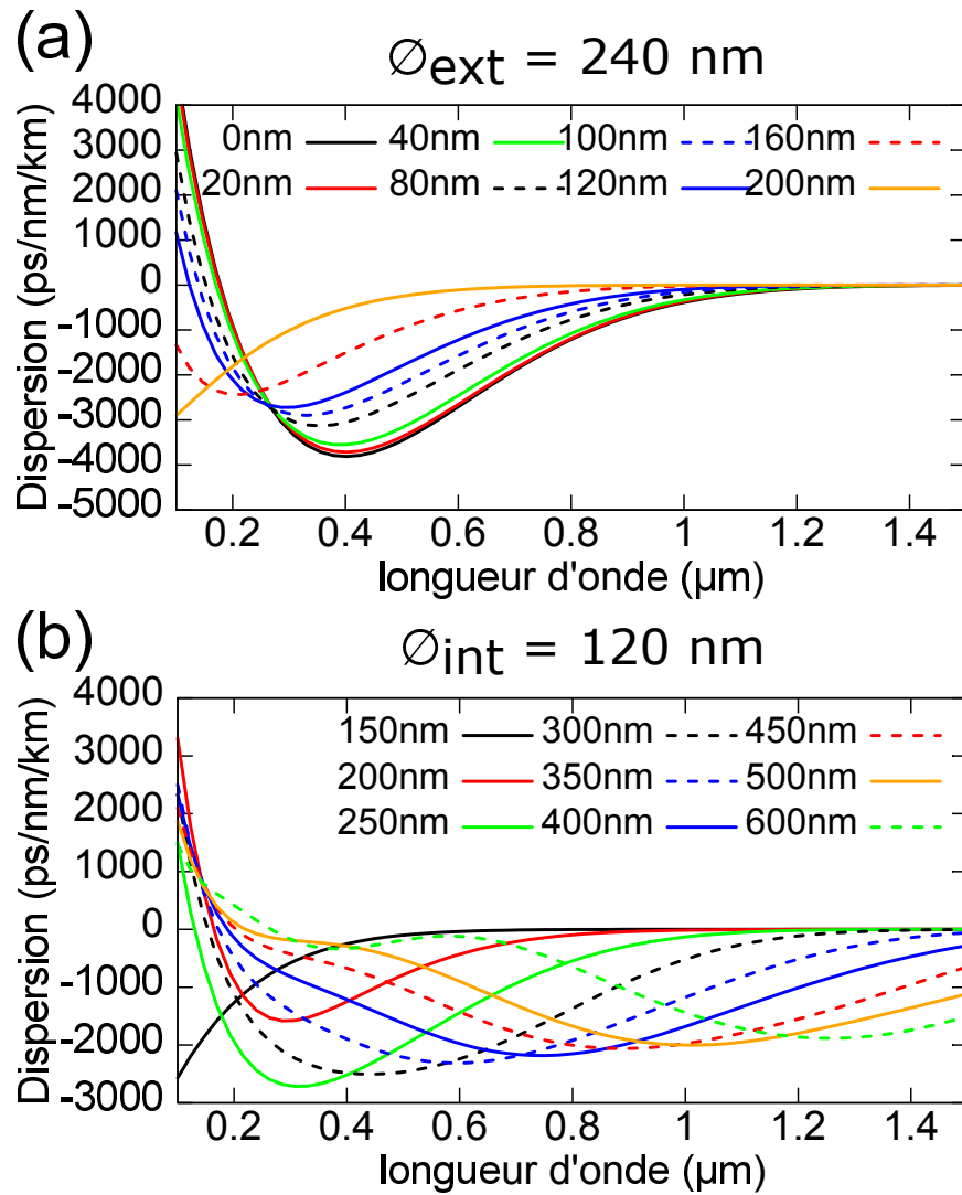
FIGURE II)-8 – Dispersion dans le cas de nanotube (a) : un diamètre externe fixé à 240 nm pour un diamètre interne variant dans la gamme [0:200] nm et (b) : un diamètre externe variant dans la gamme [150:700] nm pour un diamètre interne fixé à 120 nm.
