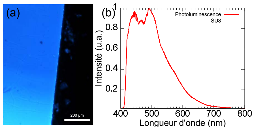
FIGURE IV)-4 – Cliché par microscopie optique d'une couche mince de SU8 exhibant une forte autofluorescence bleue sous excitation UV (a) : cliché et (b) : spectre d'émission ( \lambda = [330-380] nm, acquisition = 2 s, gain = 3,40).
