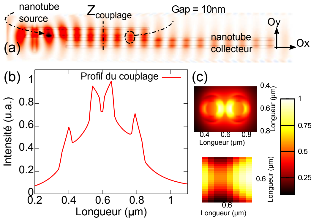
FIGURE II)-13 – Couplage optique entre nanotubes pour deux nanotubes de diamètres externe et interne respectivement de 240 nm et 120 nm, interdistants de 10 nm (a) : dans le plan (Oxy) et (b) : selon une section perpendiculaire à l'axe de propagation (Oyz) (c) : en plan large et rapproché.
