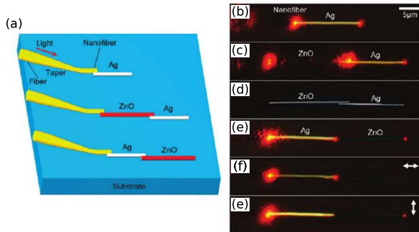
FIGURE I)-38 – (a) : Schéma des différentes méthodes de couplage entre nanofils de ZnO (guidage de photon) et d'argent (plasmon). Injection dans (b) : un nanofil de Ag, (c,d) : un nanofil de ZnO vers un nanofil de Ag, (e) : nanofil de Ag vers un nanofil de ZnO, (f,g) : suivant des polarisations parallèle et antiparallèle aux nanofils d'après [94].
