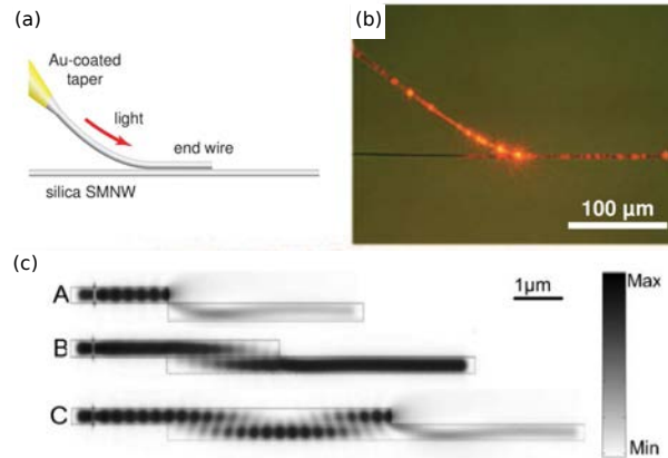
FIGURE I)-28 – Couplage évanescent entre une fibre étirée et un nanofils de silice (a) : schématisé et (b) : sous microscope optique d’après [76]. (c) : Modélisation numérique FDTD de ce couplage inter-système d’après [77].
