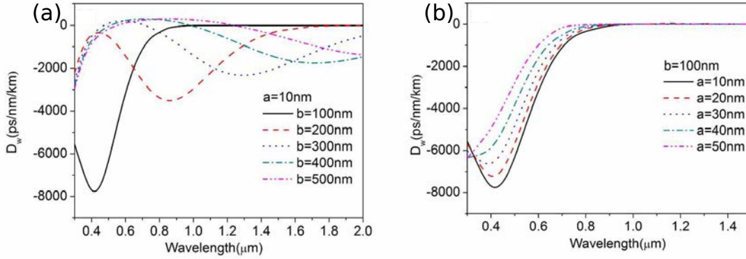
FIGURE I)-12 – Dans les cas de nanotubes dont a et b correspondant respectivement aux rayons internes et externes pour une longueur d’onde \lambda = 633 \text{ nm} , (a,b) : évolution de la dispersion modale en fonction de la longueur d’onde pour différentes valeurs de a et b d’après [21].
