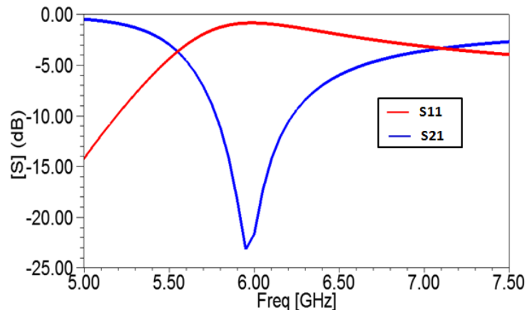
Figure 3.23. Résultats de simulation des paramètres S11 et S21 du filtre coupe bande à base des cellules CSRR rectangulaire
