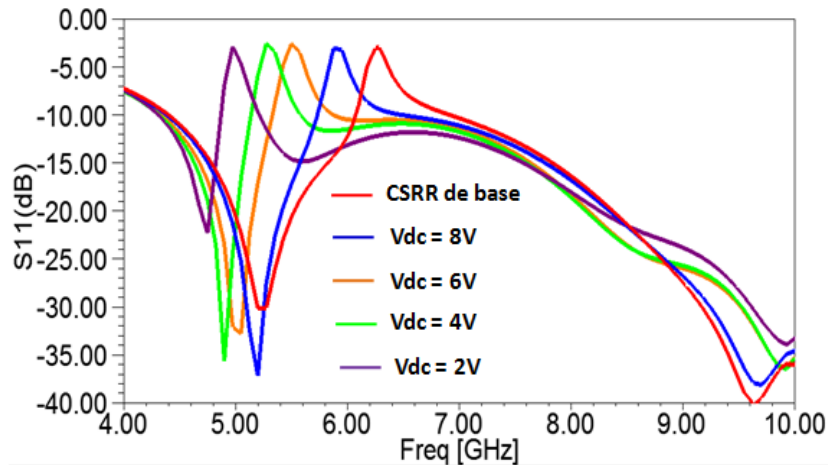
Figure 5.12. Variation du paramètre S11 en fonction de la tension Vdc de l'antenne ULB associée à un système de filtrage en amont à bande rejetée reconfigurable
