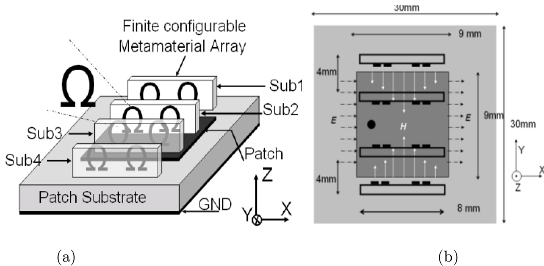
Figure 1.30. (a) Configuration de l'antenne patch associée au (SMIA) forme par un réseau fini de cellules \Omega unitaires (b) disposition et orientation des cellules \Omega en fonction des lignes de champs proche \vec{E} et \vec{H} [52]
