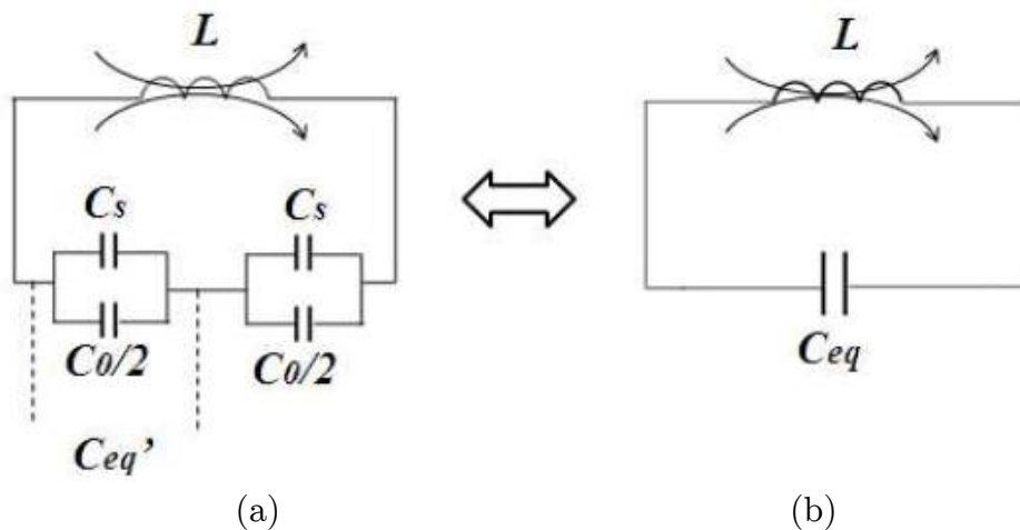
Figure 2.16. (a) modèle équivalent de la cellule SRR en fonction de L , C_s et C_0 (b) modèle équivalent simplifié en fonction de L et C_{eq}
