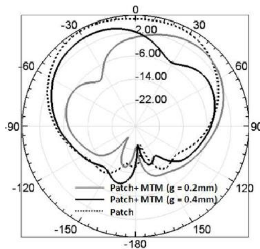
Figure 1.31. Dépointage du faisceau, en fonction des paramétrique géométriques du superstrat de l'antenne patch couverte par le superstrat SMIA [52]
