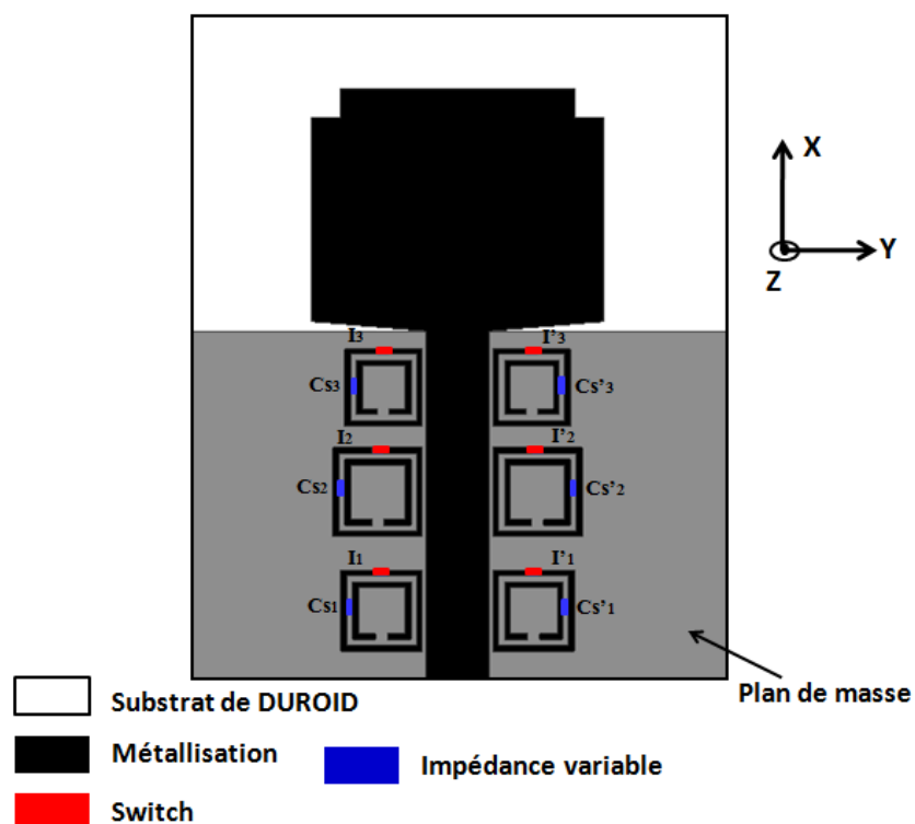
Figure 5.21 : configuration de l'antenne monopole ULB associée à trois couples de cellules SRR chargés par des couples d'interrupteurs et d'impédances capacitives
