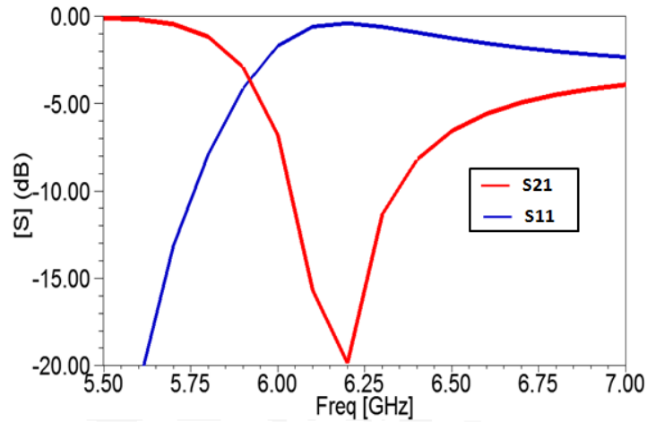
Figure 3.2. Résultats de simulation des paramètres S11 et S21 de la cellule SRR carrée
