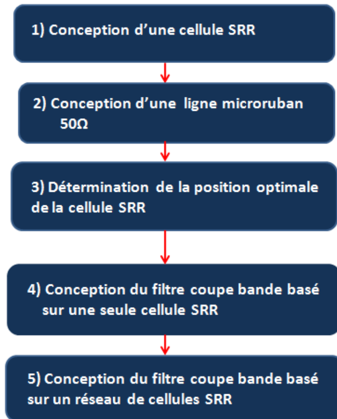
Figure 3.1. Démarche méthodologique de la conception d'un filtre coupe bande à base des cellules Métamatériaux SRR
