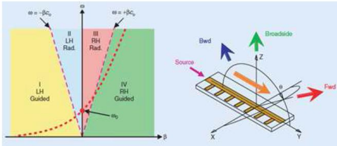
(a) (b) Figure 1.32. (a) Diagramme de dispersion d'une cellule « CRLH-TL » (b) Configuration de l'antenne (Backfire-to-Endfire Scanning Antenna) [53]
