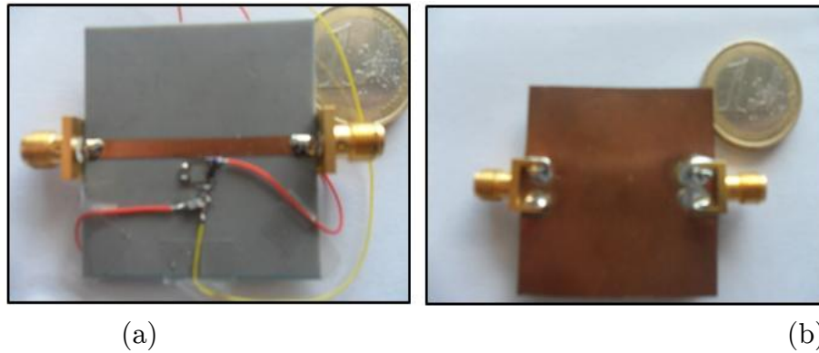
Figure 3.40. Photos de fabrication du filtre coupe bande basé sur l'association de la ligne microruban 50 \Omega à une cellule Métamatériau chargée par une diode PIN. (a) vue de dessus (b) vue de dessous
