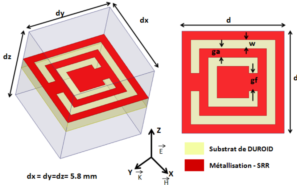
Figure 2.8. Configuration de la cellule unitaire CSRR dans sa boîte de calcul
