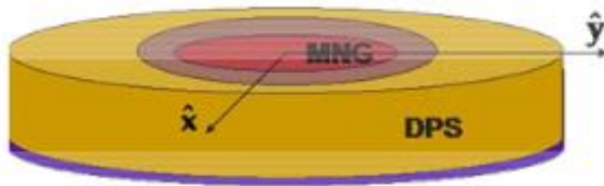
Figure 1.24. Antenne patch circulaire imprimée sur un substrat composé [33]
