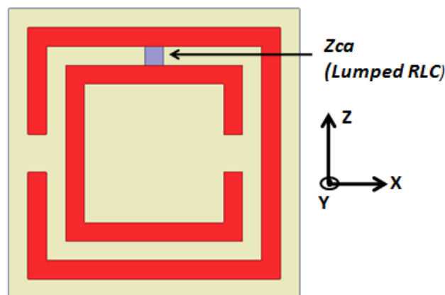
Figure 2.17. Cellule SRR chargée par une impédance Zca
