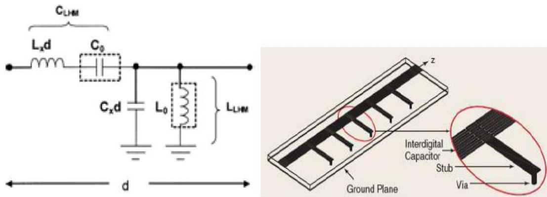
Figure 1.11. (a) modèle de la ligne CRLH-TL (b) Réalisation pratique de la ligne CRLH-TL proposée par l'équipe de T.Itoh [19]
