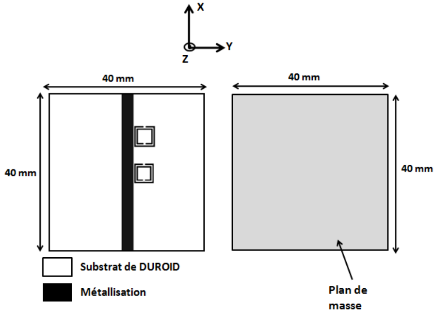
Figure 3.18 : configuration du filtre basé sur l'association de la ligne microruban 50 \Omega à deux cellules Métamateriaux SRR.
