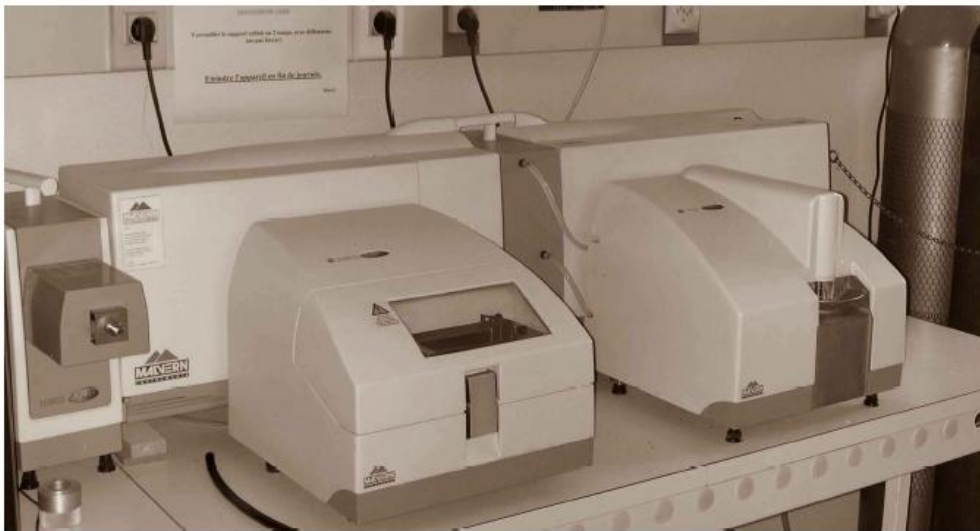
Figure 67 : Granulomètre Mastersizer 2000 _ Malvern Instrument
