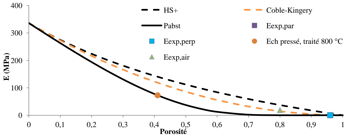
Figure 67 : Evolution du module d'Young en fonction du taux de porosité, pour un échantillon de bentonite obtenue avec une congélation lente
