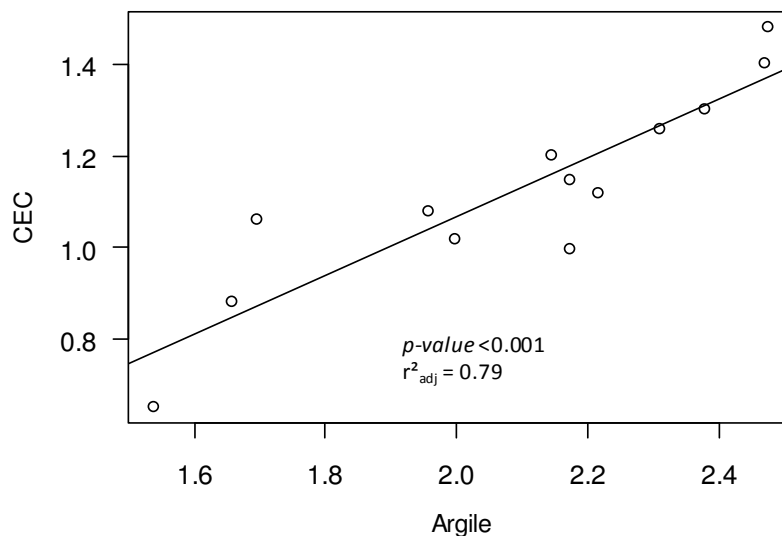
Figure 44 : Relation ente la CEC et le taux d'argile dans les sols des sites industriels d'Auzon, SHSE et de Metaleurop.
