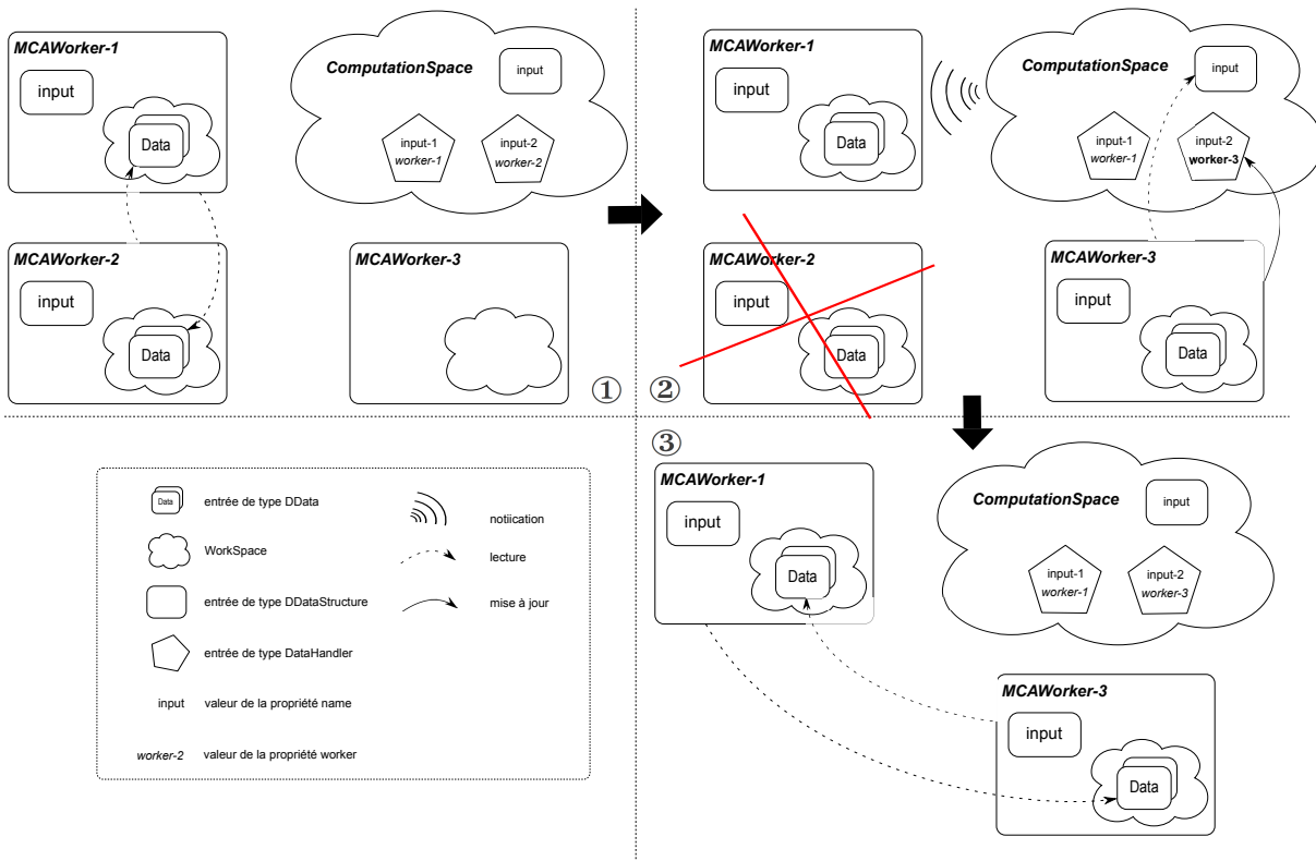
FIGURE 4.30 – Tolérance aux pannes dans les Structures de Données Distribuées. ① Partage d'une structure de données distribuées, nommée input , entre deux agents MCAWorker ( MCAWorker-1 et MCAWorker-2 ). ② Panne de l'agent MCAWorker-2 , reprise de la partie disponible ( input-2 ) par l'agent MCAWorker-3 et notification des modifications à l'agent MCAWorker-1 . ③ L'agent MCAWorker-1 peut de nouveau lire les données contenues dans la partie input-2 .
