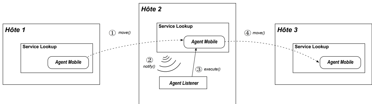
FIGURE 4.8 – Composants nécessaires à la mise en place d’un agent mobile proactif . ① L’agent mobile migre de l’Hôte 1 vers l’Hôte 2. ② L’ AgentListener est notifié de l’arrivée de l’agent mobile. ③ L’ AgentListener de l’Hôte 2 exécute le code de l’agent mobile. ④ À la fin de son exécution, l’agent mobile migre de l’Hôte 2 vers l’Hôte 3.
