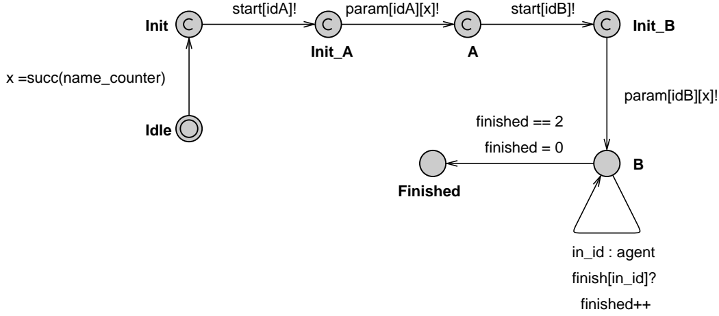
FIGURE 3.15 – Modélisation de la \pi -transformation du terme System (eq. 3.1).
