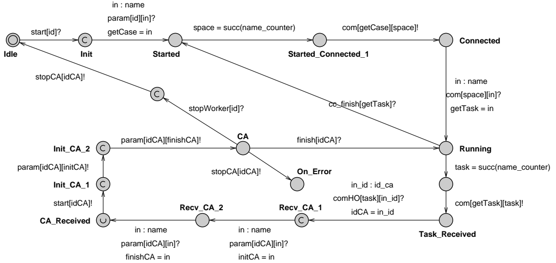
FIGURE 3.25 – Modèle d'automate Worker : résultat de la \pi -transformation du terme Worker (eq. 2.64)
