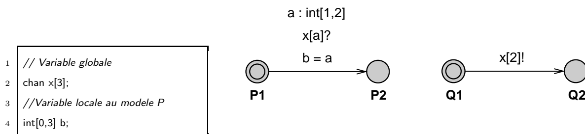
FIGURE 3.6 – Exemple d'utilisation d'une action de synchronisation non-déterministe.
