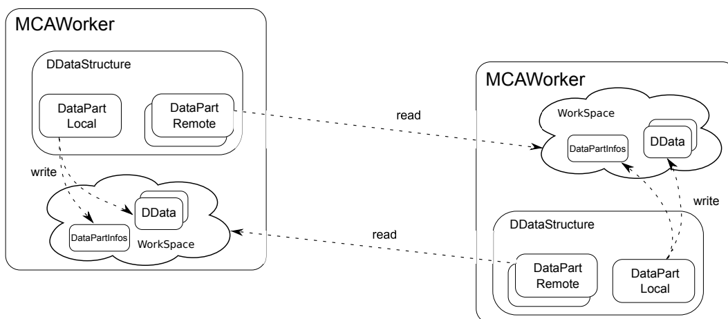
FIGURE 4.27 – Communication entre deux parties d'une Structure de Données Distribuée.
