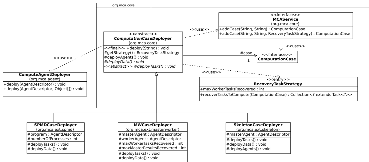
FIGURE 5.10 – Diagramme des classes utilisées lors du déploiement d'un cas de calcul sur la plate-forme MCA .
