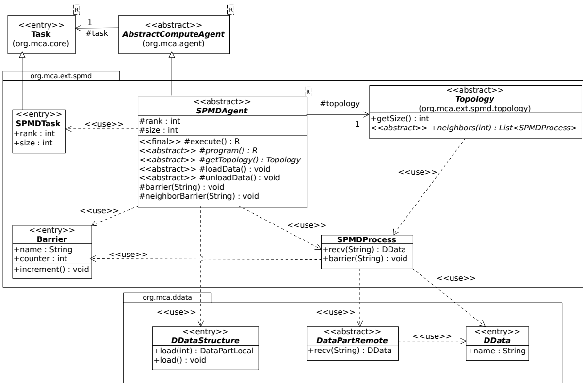
FIGURE 5.12 – Diagramme de classe de l’API MCA-SPMD
