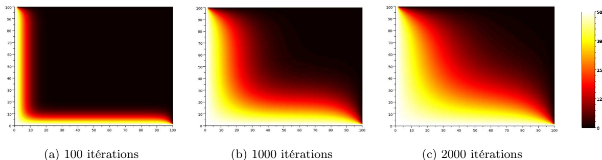
FIGURE 5.15 – Visualisation à l'aide de l'outil Scilab de l'évolution de la température avec la résolution de l'équation de Laplace dans le plan en fonction du nombre d'itérations.
