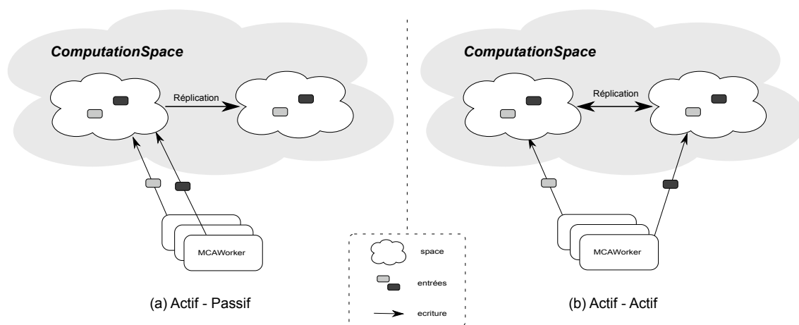
FIGURE 4.12 – Les deux types de topologies possibles au sein d'un ComputationSpace défini comme un groupe de réplication.
