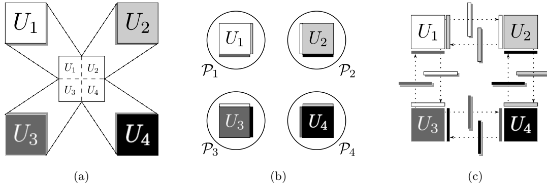
FIGURE 5.16 – Modélisation d’une itération de Jacobi parallèle sur 4 processus : (a) partage de la matrice en sous-matrices ( U_1, U_2, U_3 et U_4 ); (b) chaque processus ( \mathcal{P}_1, \mathcal{P}_2, \mathcal{P}_3 et \mathcal{P}_4 ) reçoit une sous-matrice ainsi que les bords des sous-matrices voisines. (c) : à chaque itération les bords sont mis-à-jour et sont échangés avec les processus qui traitent les sous-matrices voisines.
