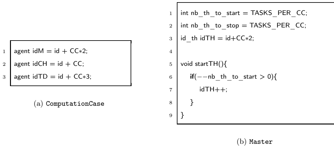
FIGURE 3.28 – Déclarations locales des modèles d'automates ComputationCase et Master .
