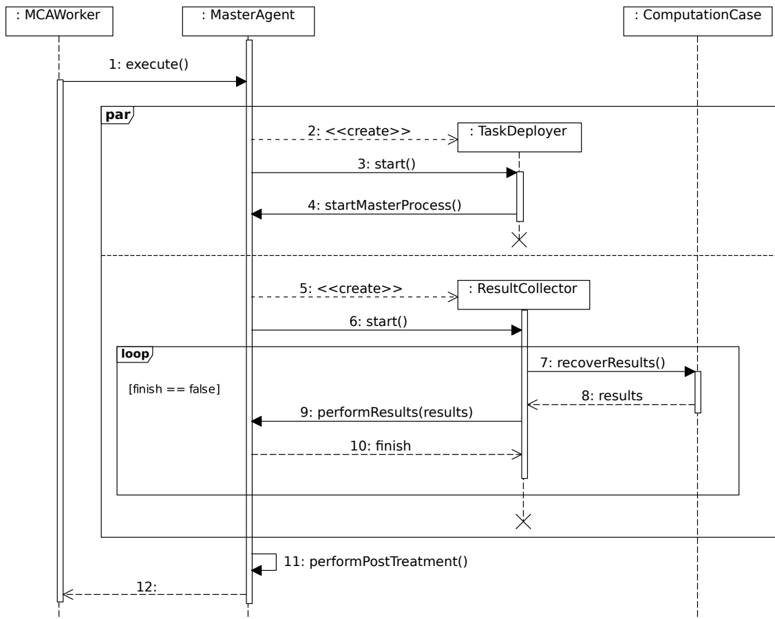
FIGURE 5.21 – Diagramme de séquence de l’exécution générique d’un agent de type MasterAgent .
