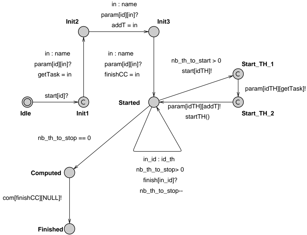
FIGURE 3.27 – Modèle d'automate Master : résultat de la \pi -transformation du terme Master (eq. 3.7)
