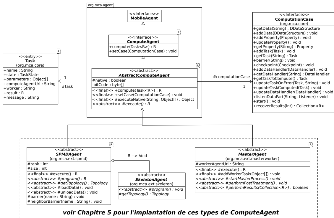
FIGURE 4.23 – Diagramme des classes utilisées pour définir un ComputeAgent .
