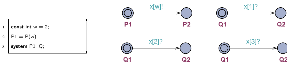
FIGURE 3.5 – Déclaration d'un système UPPAAL de quatre automates temporisés.
