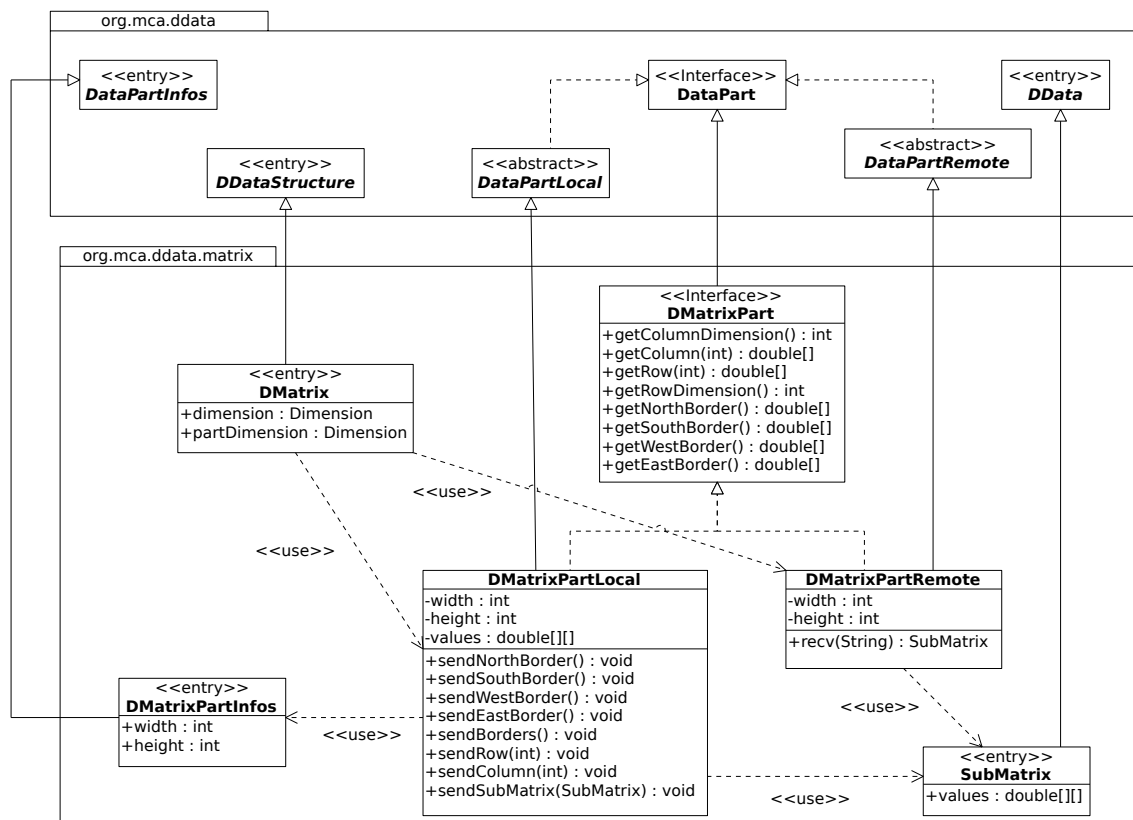
FIGURE 4.28 – Diagramme des classes pour la manipulation d'une matrice distribuée.
