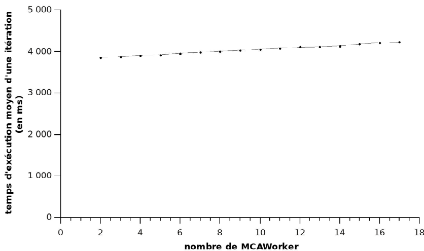
FIGURE 5.18 – Adaptabilité de la plate-forme MCA en fonction du nombre d'agents MCAWorker
