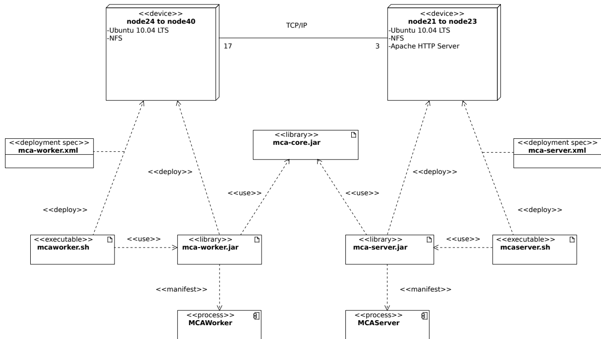
FIGURE 5.2 – Diagramme de déploiement des composants MCA Worker et MCA Server sur la grille de calcul du LACL.
