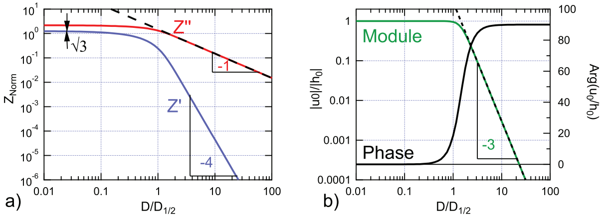
FIGURE 2.11 – Résultat de la résolution numérique de l'équation élasto-hydrodynamique pour une couche mince incompressible sur un plan infiniment rigide. (a) : Impédance hydrodynamique normalisée ( Z_{Norm} = Z \times D_{1/2}/4\pi\eta\omega R^2 ) en fonction de la distance sphère-plan D normalisée par la distance de coupure D_{1/2} . À grande distance, la dissipation visqueuse Z'' retrouve la loi de Reynolds, tandis que la partie élastique Z' varie comme D^{-4} . À fort confinement ( D \ll D_{1/2} ) l'impédance hydrodynamique sature et le rapport partie visqueuse sur élastique tend vers \sqrt{3} . Cette courbe est en théorie adaptable à tout système film mince compressible sur plan infiniment rigide : la correspondance avec un système réel se fait par simple translation de la courbe ici représentée dans un diagramme log-log, ce qui détermine la distance de coupure D_{1/2} et donc le module d'Young E du film (si l'on connaît les autres paramètres dont dépend D_{1/2} ). (b) : Indentation maximale du film (sur l'axe de symétrie du système) en fonction de la distance normalisée. À faible confinement |u_0| varie comme D^{-3} et est en quadrature de phase avec l'oscillation de la sphère. À fort confinement |u_0| = |h_0| : le liquide est localement clampé entre la sphère et le plan.
