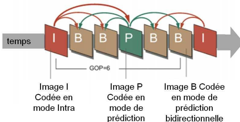
FIGURE 34. Groupe d'images GOP : dans cet exemple, le rassemblement est de type IBBPBI.
