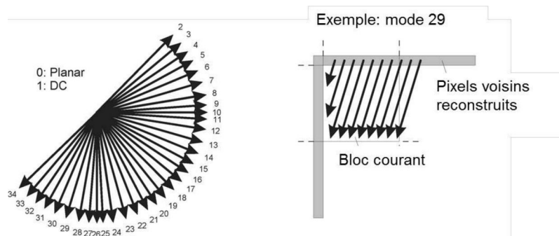
FIGURE 40. 33 directions possibles de prédiction Intra dans HEVC.
