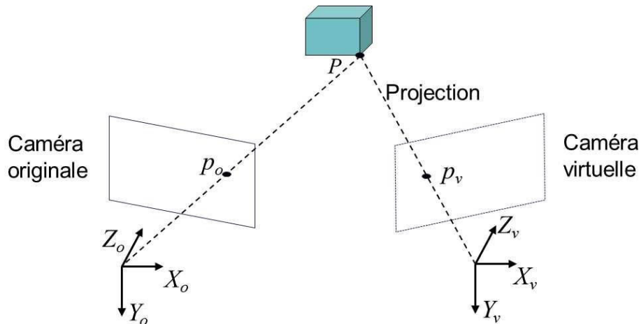
FIGURE 23. Synthèse de vue virtuelle par projection d'un point P du plan de la caméra originale sur le plan de la caméra virtuelle.
