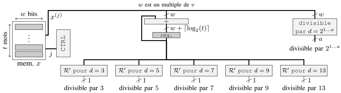
FIGURE 5.4 – Architecture des tests de divisibilité par \mathcal{D} = (2^{1\dots a}, 3, 5, 7, 9, 13) en utilisant l'amélioration en base 2^v des rubans de Pascal.
