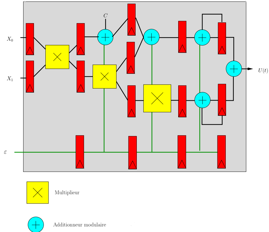
FIGURE 1.9 – Unité arithmétique contenue dans un Rowser pour ECC (source [54]).
