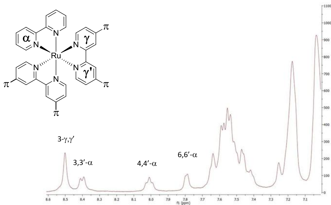
Figure 83 : Partie aromatique du spectre RMN 1 H du composé 5 dans le CD 2 Cl 2 .
