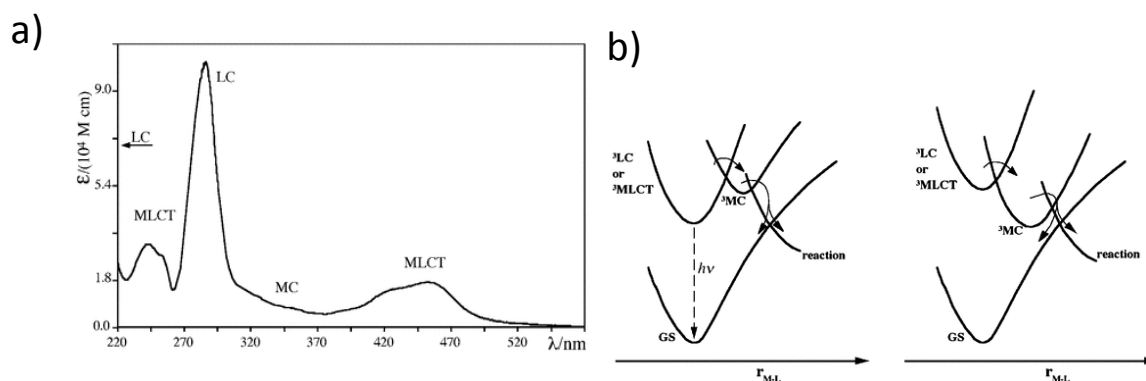
Figure 7 : a) Spectre d'absorption de \text{Ru}(\text{bpy})_3\text{Cl}_2 dans l'éthanol ; b) représentation schématique des deux cas limites de la position de la transition ^3\text{MC} par rapport aux autres transitions 1 .
