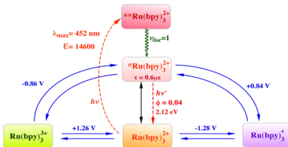
Figure 8 : Processus photo-physiques et électrochimiques des différents états excités ainsi que des divers états d'oxydation de [\text{Ru}(\text{bpy})_3]^{2+} . Les différentes données spectroscopiques et les potentiels électrochimiques sont indiqués. Potentiels électrochimiques mesurés dans l'eau vs SCE 1 .
