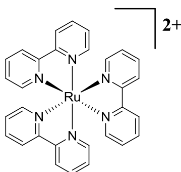
Figure 6 : Structure chimique de [\text{Ru}(\text{bpy})_3]^{2+} .
