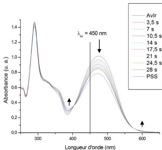
Figure 132 : Evolution du spectre d'absorption du complexe RuLa dans le Me-THF sous irradiation lumineuse à 450 nm.
