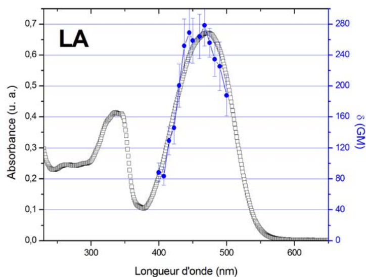
Figure 123 : Spectre d'absorption à 1 et 2 photons dans le \text{CH}_2\text{Cl}_2 à température ambiante.
