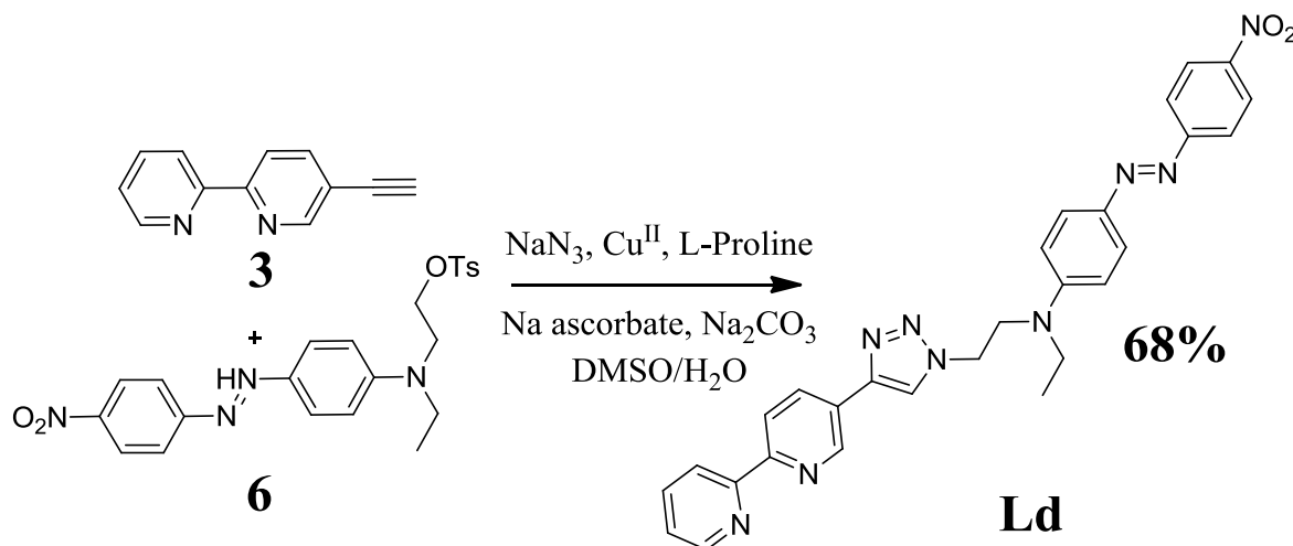
Figure 109: Synthèse du ligand Ld .
