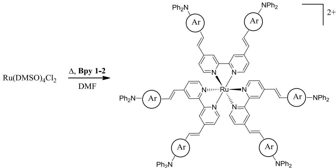
Figure 80 : Méthode de synthèse des complexes de type \text{Ru}(\text{Bpy})_3(\text{PF}_6)_2 .
