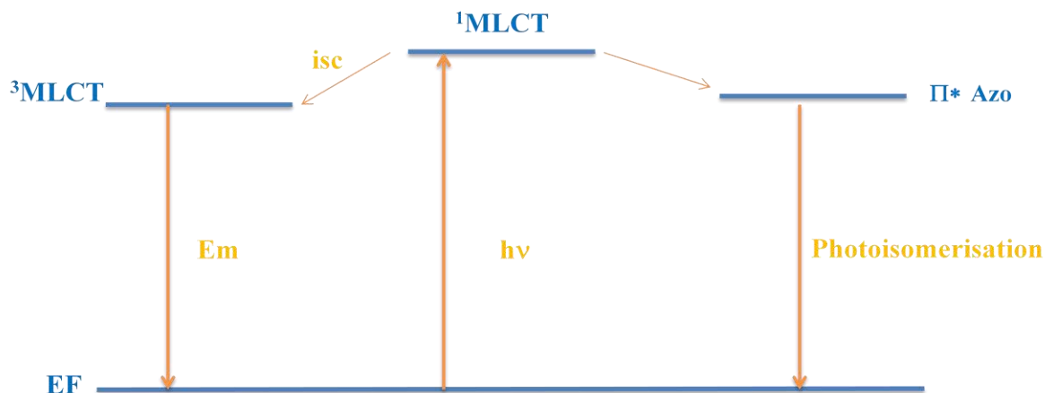
Figure 131 : Représentation des niveaux d'énergies \pi_{\text{azo}}^* et \pi_{\text{ppy}}^* ainsi que des processus photo-physiques associés.
