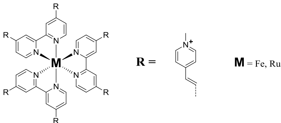
Figure 34 : Représentation des complexes étudiés par B. J. Coe et. al.
