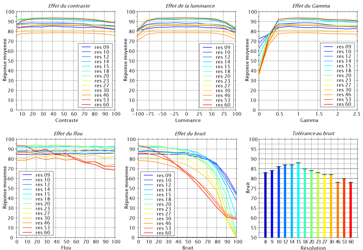
Figure III-31 Tolérance aux transformations photométriques (pour chacune des résolutions)
