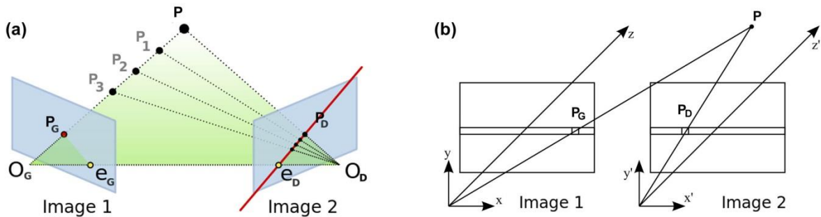
Figure II-15 Géométrie épipolaire : (a) l'ensemble des points entre le centre optique O_G et le point P se projettent dans l'image 1 au niveau de P_G et le long d'une droite correspondant à l'intersection entre le plan de l'image 2 et celui défini par les points P , O_G et O_D ; (b) en géométrie rectifiée, les projections d'un point de l'espace sur chaque image se trouvent nécessairement sur la même ligne.
