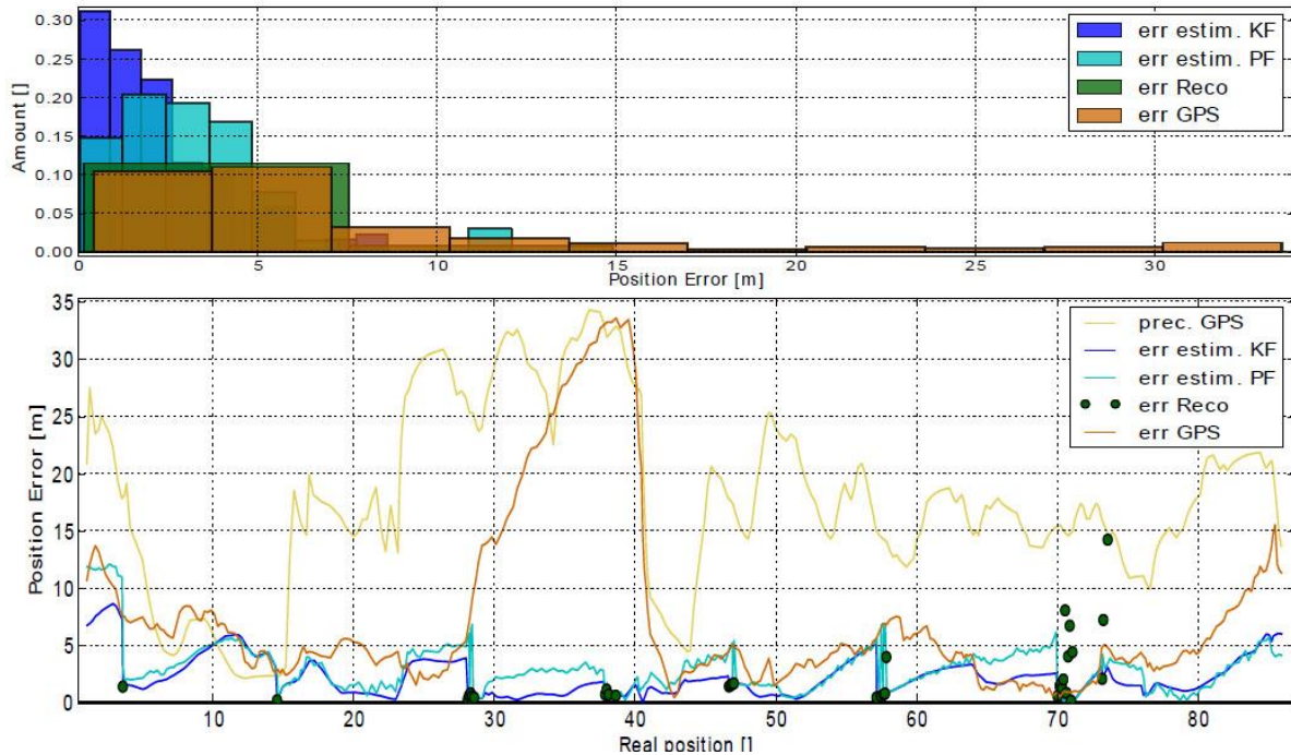
Figure II-40 Comparaison de l'erreur du filtre à particules (en turquoise) et du filtre de Kalman (en bleu)
