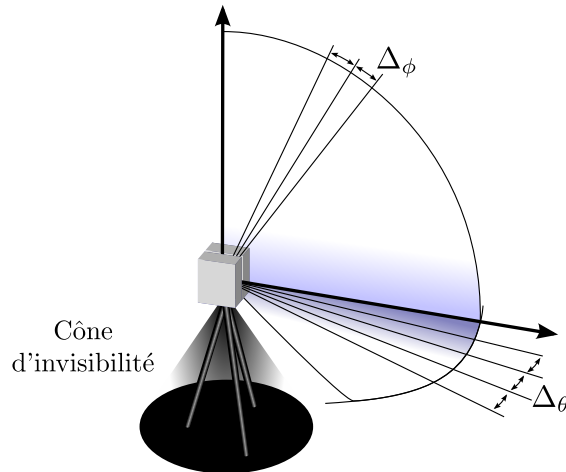
FIGURE 2.9 – Mode d'acquisition d'un laser fixe sur trépied.
