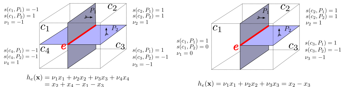
FIGURE 8.13 – Calcul des poids \nu(c, e) et de la fonction h_e(\mathbf{x}) .
