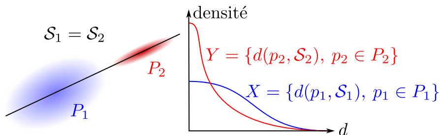
FIGURE 7.2 – Cas où \mathcal{S}_1 = \mathcal{S}_2 , X et Y sont définis par les équations (7.11) et (7.12). Les tests rejettent l'hypothèse H_0 .
