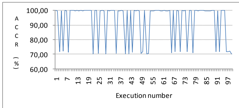
m=6
