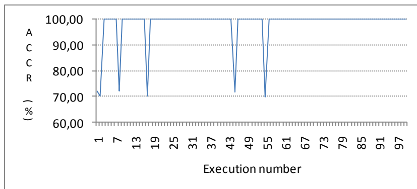
m=4
