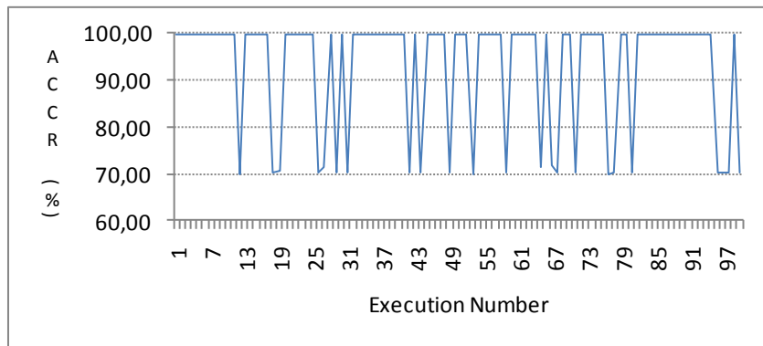
m=2
