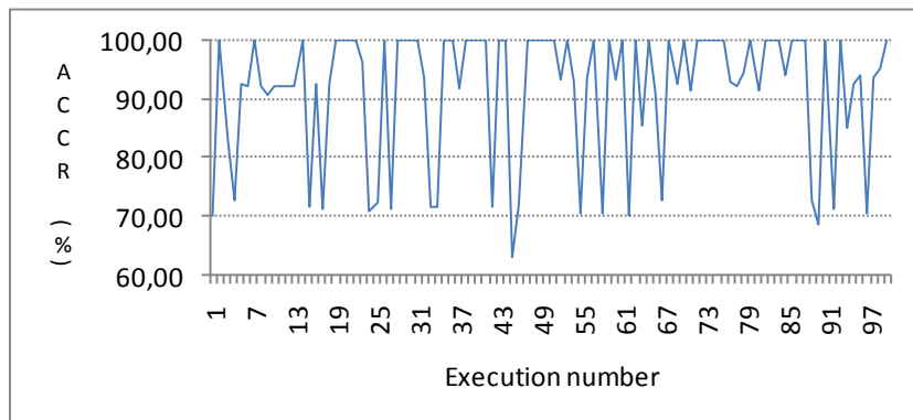
m=8
