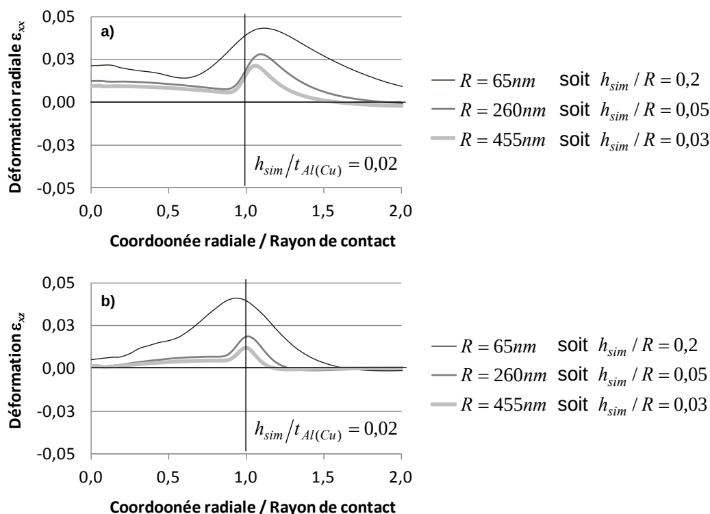
Figure V-49 – Evolution de la déformation élastique a) radiale selon l'axe x ( \varepsilon_{xx} ) et b) de cisaillement ( \varepsilon_{xz} ), en fonction de la coordonnée radiale pour un rapport d'enfoncement ( h_{sim} ) sur épaisseur de film d'Al(Cu) ( t_{Al(Cu)} ) de 2%, à la surface du film d'Alumine native, pour des rugosités de Nickel de rayon 65, 260 et 455nm.
