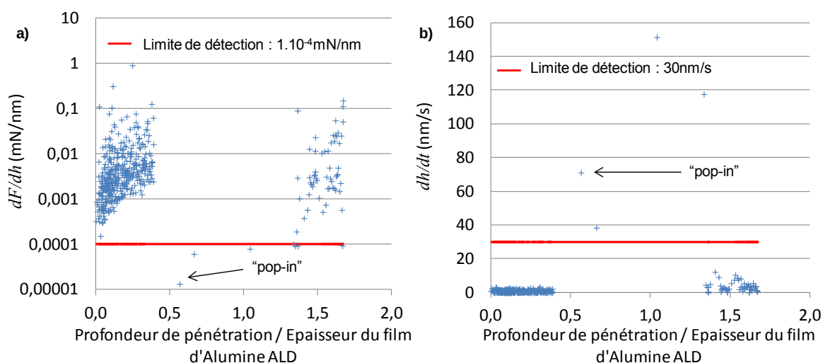
Figure IV-60 – Evolutions des pentes locales des courbes a) charge-déplacement et b) déplacement-temps en fonction de la profondeur de pénétration sur l'épaisseur d'Alumine, pour un essai d'indentation sphérique (rayon 0,45\mu\text{m} ) sur de l'Alumine ALD épaisse de 40\text{nm} .
