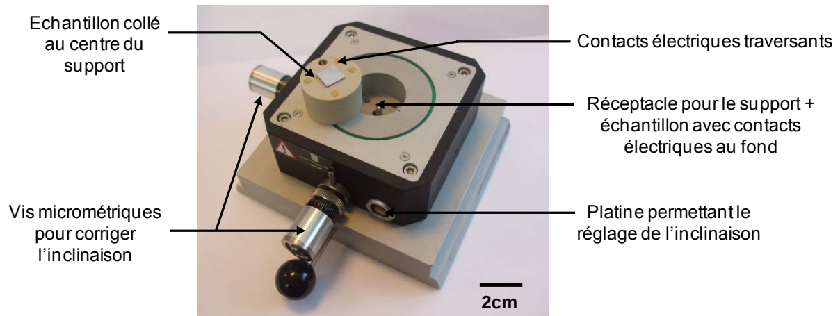
Figure III-31 – Platine inclinable et plot avec l'échantillon collé dans le cas d'une microinsertion avec mesure électrique.
