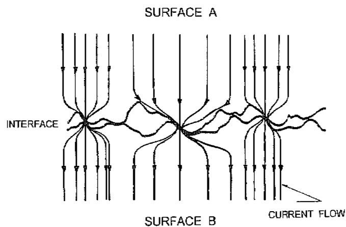
Figure II-30 – Représentation schématisée d'une interface électrique entre matériaux massifs [SLADE 1999].
