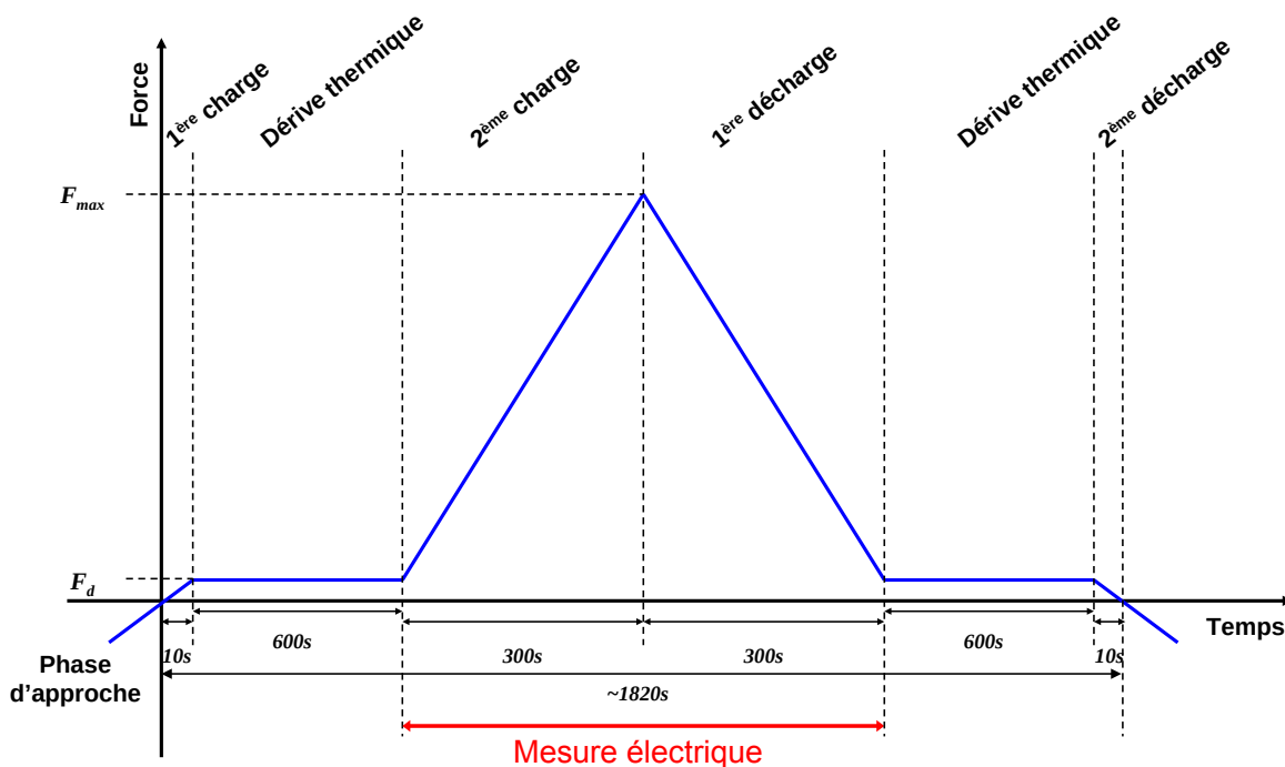
Figure III-38 – Protocole expérimental pour l'essai d'insertion avec mesure électrique.
