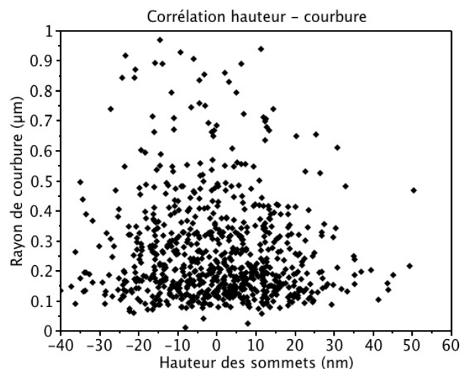
Figure IV-28 – Graphique représentant la distribution des rayons de courbure en fonction des hauteurs des sommets de chaque aspérité.
