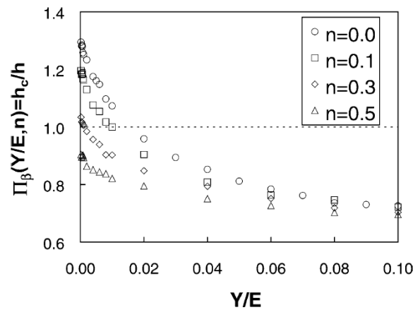
Figure III-12 – Relations entre h_c/h et Y/E pour différentes valeurs de coefficients d'érouissage n , avec Y la limite élastique du matériau [CHENG 2004].
