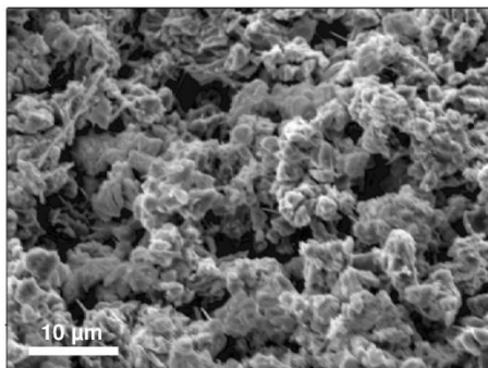
Figure II-33. Image MEB de la surface de l'électrode V, après une capacité lithiée de 3700 mAh.g -1 .
