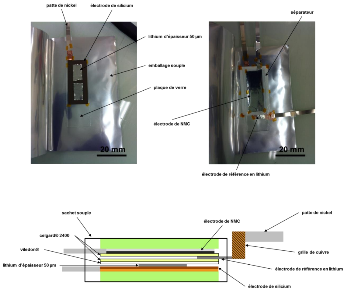
Figure IV-21. Photographies de l'assemblage et schéma du montage d'un accumulateur Li-ion contenant une électrode négative de silicium et de lithium.
