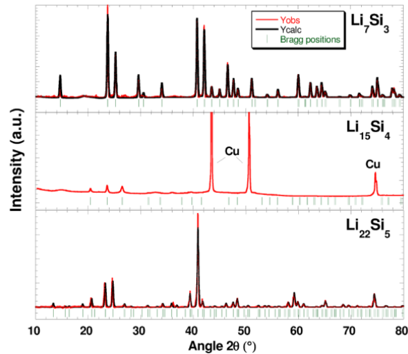
Figure II-9. Diffractogrammes obtenus pour \text{Li}_7\text{Si}_3 , \text{Li}_{15}\text{Si}_4 et \text{Li}_{22}\text{Si}_5 .
