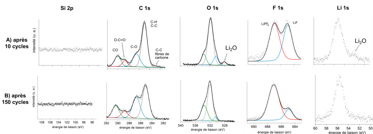
Figure IV-7. Spectres XPS Si 2p, C 1s, O 1s, F 1s et Li 1s obtenus à la surface des électrodes cyclées sur 1200 \text{mAh}\cdot\text{g}^{-1} dans le domaine \beta , A) après 10 cycle, B) après 150 cycles. Les analyses ont été réalisées en fin de lithiation, i. e. lorsque le potentiel atteint 0,005 V.
