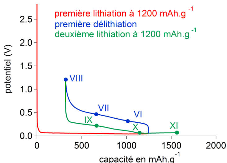
Figure II-44. Courbes de potentiel d'une pile bouton constituée d'une électrode de silicium micrométrique face à du lithium métal cyclée à un régime de C/20 dont la capacité en lithiation (ou décharge) est bloquée à 1200 mAh.g -1 . Les électrodes analysées par AES (IX, X et XI) sont représentées par des points verts.
