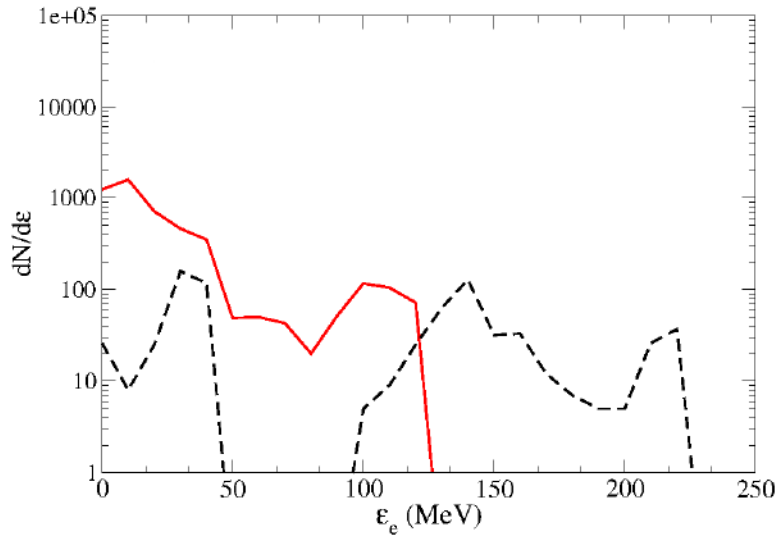
Figure 4.19: Effet des pertes par rayonnement sur les distributions en énergie des électrons à t = 100T_L : distribution en énergie des électrons pour l = 1/8\lambda_L et n_e = 100n_c . La ligne rouge représente les cas avec prise en compte de la réaction du rayonnement. Les pertes par rayonnement ne sont pas considérées pour le cas illustré par des tirets noirs.
