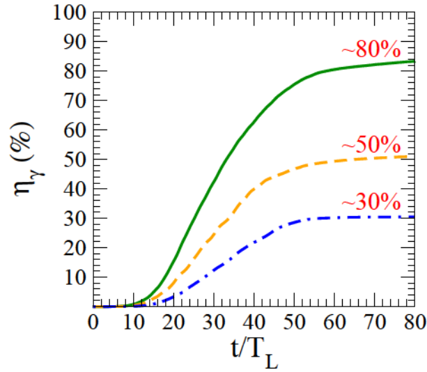
Figure 5.20: Énergie rayonnée \eta_\gamma en fonction du temps dans le cas d'un plasma épais d'ions et d'électrons. En trait vert: plasma d'ions immobiles. En pointillés oranges: plasma de deutérons. En pointillés et tirets bleus: plasma de protons. a_0 = 200 et n_{e0} = 10n_c . La durée de l'impulsion laser est de 14 T_L .
