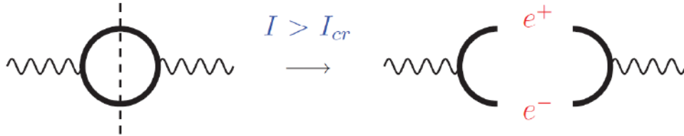
Figure 2.13: Production de paires par la “cassure” de la polarisation du vide. Les lignes oscillantes représente les photons se propageant dans le vide. Le cercle noir (a) représente les fluctuations quantiques du vide composées de paires particule-antiparticule. Cette fluctuation interagit avec le champ extérieur (b), pour I \geq I_{cr} engendrant une création réelle de particule-antiparticule.
