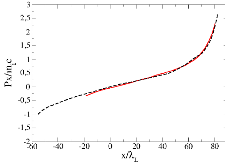
Figure 4.18: Effet de la réaction du rayonnement sur l'espace des phases des ions à t = 100T_L : pour une densité de 10n_c avec une épaisseur de 1/8\lambda_L . En traits rouges: avec prise en compte des pertes par rayonnement. En tirets noirs: sans prise en compte des pertes par rayonnement.
