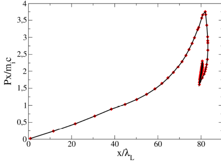
Figure 4.4: Espace des phases des ions à t = 100T_L . n_e = 100n_c et l = 0.5\lambda_L . I = 5.1 \times 10^{22} \text{W/cm}^2 . Le laser est polarisé circulairement. Avec pertes radiatives (points noirs) et sans pertes radiatives (ligne rouge).
