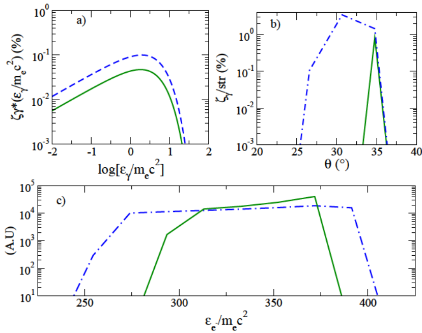
Figure 4.33: Spectre en énergie du faisceau d'électrons et des photons émis pour a_0=200 et \gamma_0=100 , avec pertes par rayonnement au temps où l'énergie cinétique du faisceau est maximale. En pointillés bleus: avec un profil trapézoïdal. En traits verts: avec un profil gaussien.
