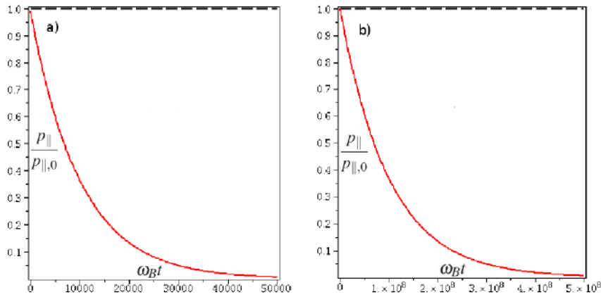
Figure 2.9: p_{\parallel}/p_{\parallel,0} fonction de \omega_B t . (a): B=10^9\text{T} et \gamma=100 . (b): B=10^5\text{T} et \gamma=1000 . En trait rouge: avec la considération des pertes par rayonnement. En pointillés noirs: sans la considération des pertes par rayonnement.
