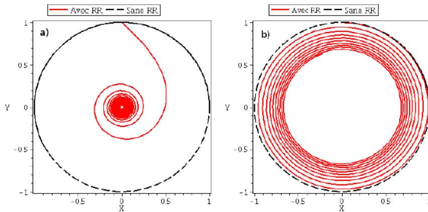
Figure 2.10: Orbite de l'électron dans le plan (X,Y) , perpendiculaire à \mathbf{B} . (a): B=10^9\text{T} et \gamma=100 . (b): B=10^5\text{T} et \gamma=1000 . Les axes sont normalisés au rayon de Larmor initial de l'électron. En trait rouge: avec la considération des pertes par rayonnement. En pointillés noirs: sans la considération des pertes par rayonnement.
