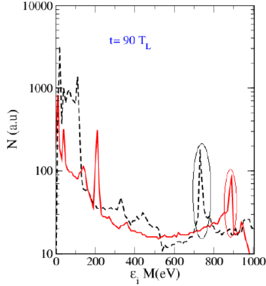
Figure 4.13: Spectre en énergie des ions à t = 90 T_L . En traits rouges: avec pertes par rayonnement. En pointillés noirs: sans pertes par rayonnement.
