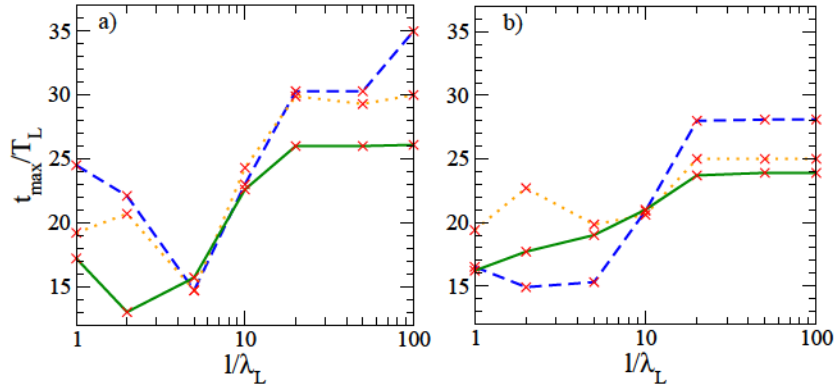
Figure 5.10: Dépendance de t_{\max} en fonction de l'épaisseur de la cible plasma, l ; (a): laser polarisé circulairement; (b): laser polarisé linéaire. En pointillés bleus: plasma de protons. En points orange: plasma de deutérons. En trait vert: plasma d'ions immobiles.
