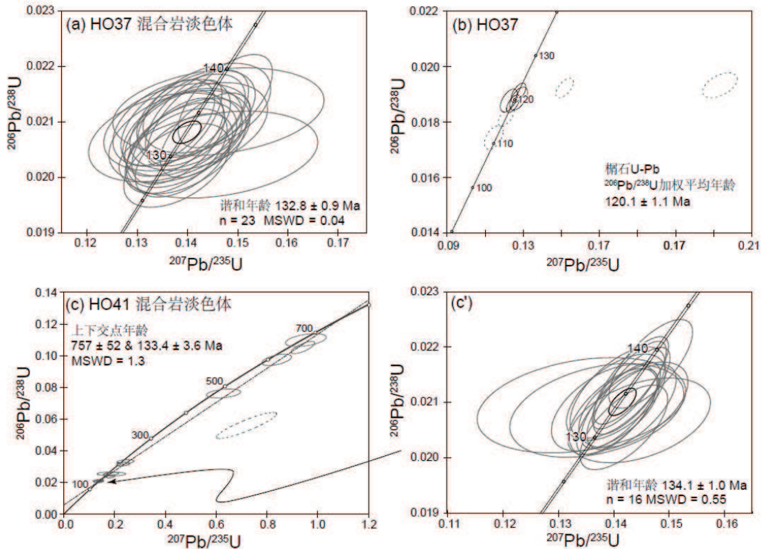
图 3-9 桐柏杂岩混合岩浅色体锆石和榍石 U-Pb 年龄谐和图
