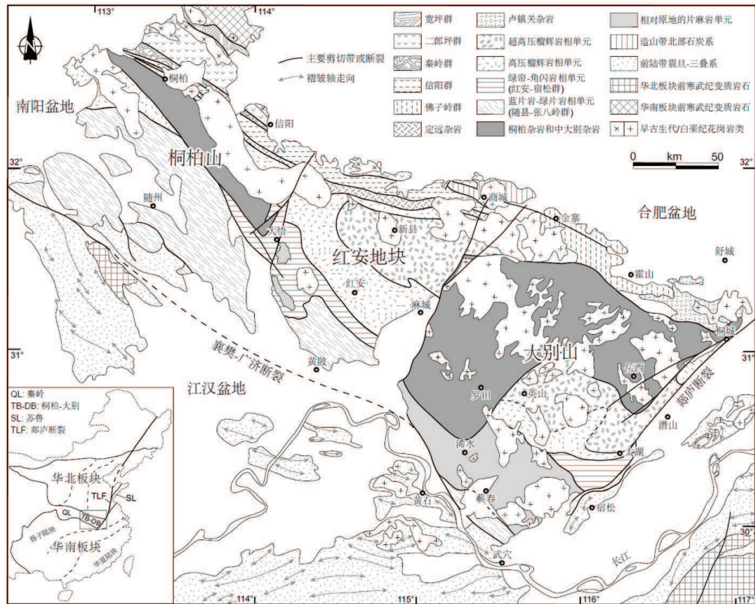
图 3-2 桐柏-大别造山带构造简图
