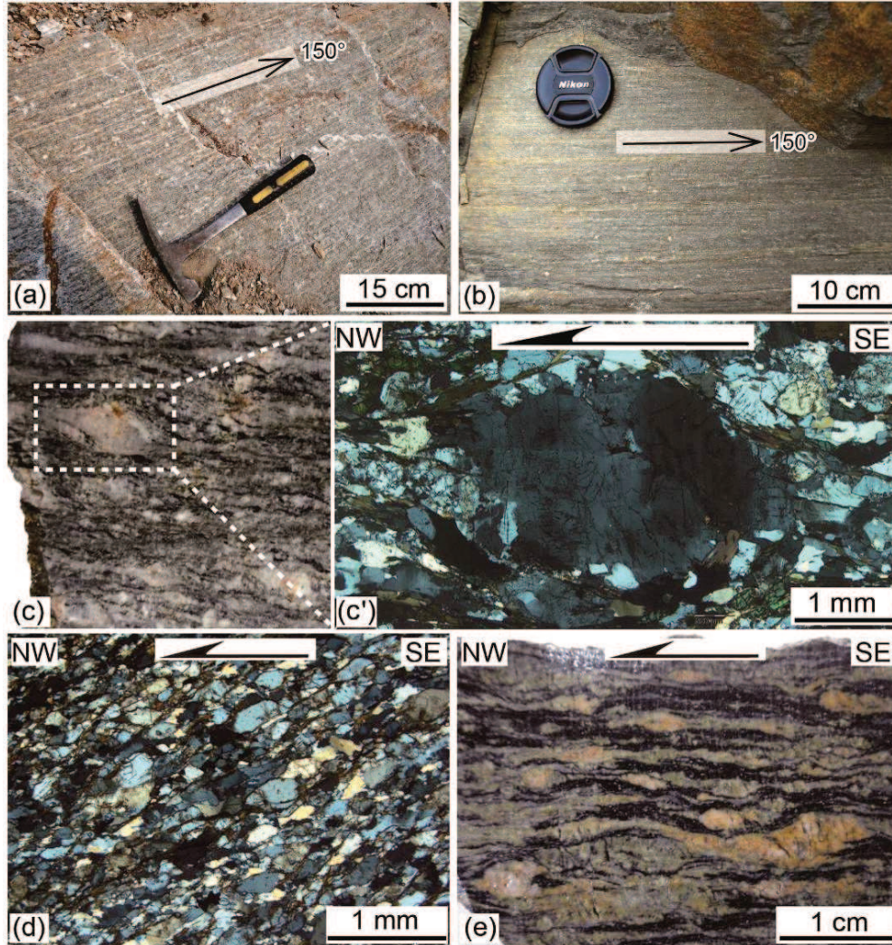
图3-22 浉水剪切带构造变形特征
