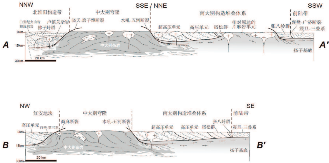
图3-16 大别山剖面示意图(位置见图3-15)
