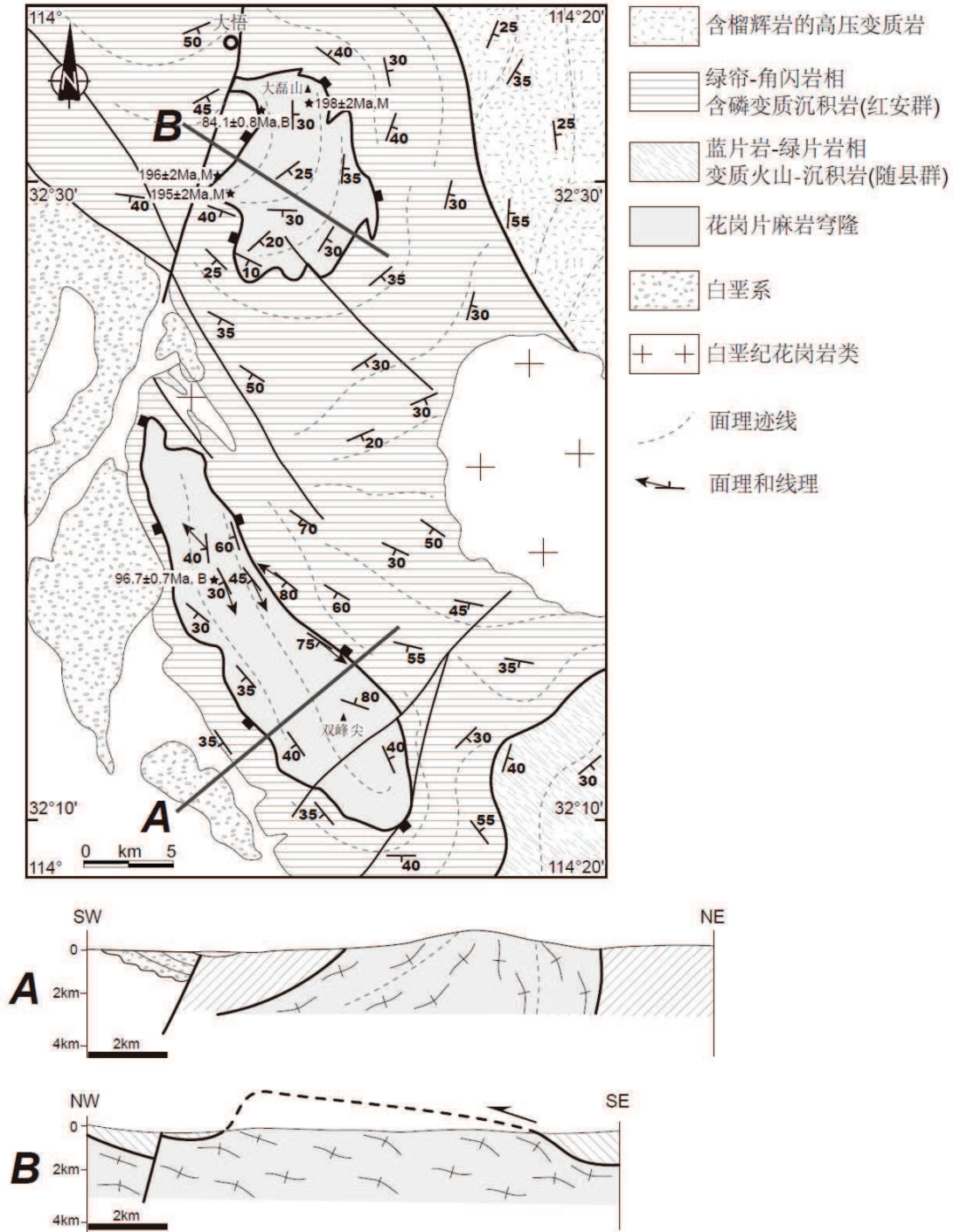
图 3-11 双峰尖和大磊山地质构造简图及构造剖面图
