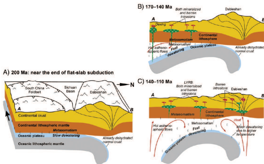
图2-4 平板俯冲模式(引自X.H. Li et al., 2013)
