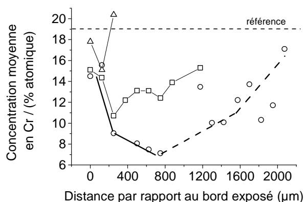
Figure IV- 14 : Evolution de la concentration (apparente) en chrome dans le film de peinture au cours du temps d'immersion dans NaCl 0,5M et selon la distance par rapport au bord exposé. (Δ) 1 jour d'immersion ; (□) 3 jours d'immersion ; (○) 6 jours d'immersion (volume d'électrolyte 20mL).
