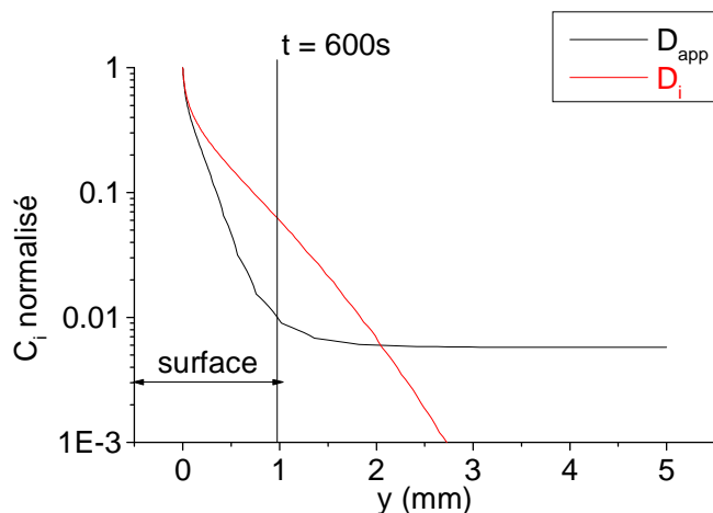
Figure V- 5 : Concentration en inhibiteurs atteinte à t= 600 secondes en régime de diffusion pure ( D_i ) et de diffusion convective ( D_{app} ).
