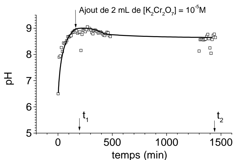
Figure III- 16 : Variation du pH à la surface d'un alliage 2024 - Mise en évidence de l'effet de l'ajout de dichromates. La solution dans la cellule après ajout des dichromates est une solution à 3.10^{-6}M et son pH nominal est de 6.65 (voir Tableau III- 1 ci-après).
