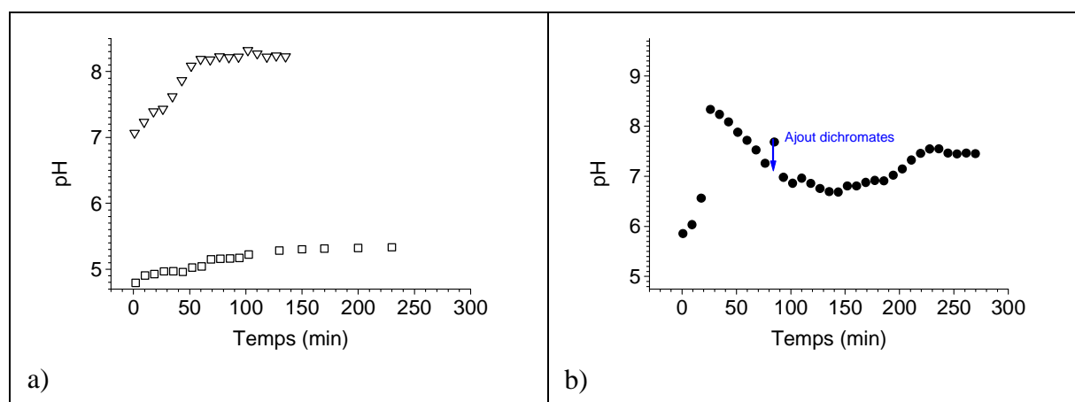
Figure III- 49 : Evolution du pH à la surface d'une solution solide Al33%atCu- Décapage au préalable 15 s dans NaOH 0.5mM ; (a) (∇) NaCl 0,1M (pH = 6.5) ; (□) NaCl 0,1M+ K_2Cr_2O_7 10^{-4}M (pH = 5,75) ; (b) (●) NaCl 0,1M + Ajout de 0,2 mL d'une solution de dichromates (concentration globale de 3.10^{-4}M (pH=5,66). Décapage initial 15s dans NaOH 0,5mM.
