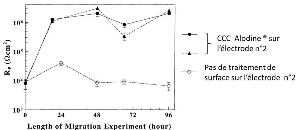
Figure I- 45 : Mesure de la résistance de polarisation d'un alliage 2024 dans NaCl 0.1M après différents temps d'exposition dans la cellule « artificial scratch cell » [56] Il est important de noter que chaque point correspond à un essai unique.
