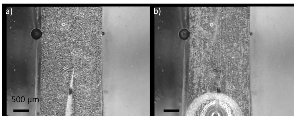
Figure III- 17 : Observation de l'échantillon # 2 (2024+OAC-Sc) a) t_1 = 3h39 (ajout des dichromates), b) t_2 = 24h . (Les temps sont indiqués sur la Figure III- 16).
