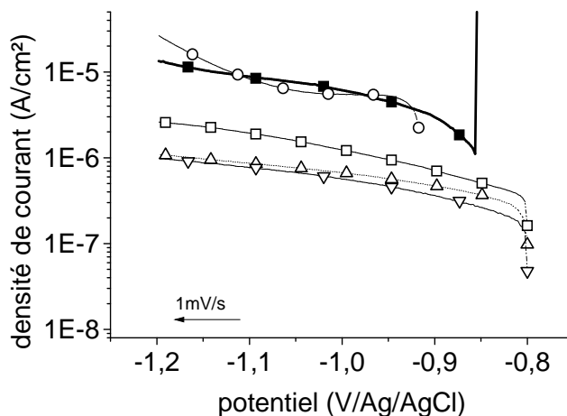
Figure III- 56 : Etude paramétrique du domaine d'efficacité des dichromates pour Al2%Cu Décapage au préalable 15 s dans NaOH 0.5mM (■) NaCl 0,1M ;(○) NaCl 0,1M + K_2Cr_2O_7 10^{-5}M ;(△) NaCl 0,1M + K_2Cr_2O_7 5.10^{-5}M ;(▽) NaCl 0,1M + K_2Cr_2O_7 10^{-4}M ;(□) NaCl 0,1M + K_2Cr_2O_7 10^{-3}M .
