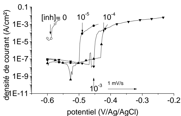
Figure III- 40 : Courbe de polarisation anodique pour une solution solide Al2%atCu dans NaCl 0,1 M et dans une solution contenant des dichromates ( 10^{-5} , 10^{-4} , 10^{-3} M) ; (○) NaCl 0,1M ; (●) NaCl 0,1M + K_2Cr_2O_7 10^{-5} M ; (▲) NaCl 0,1M + K_2Cr_2O_7 10^{-4} M ; (▼) NaCl 0,1M + K_2Cr_2O_7 10^{-3} M.
