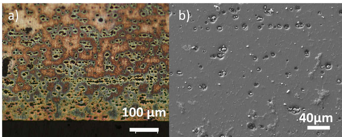
Figure III- 4 : a) Faciès d'attaque observé à potentiel libre sur un alliage 2024 immergé dans une solution NaCl 0,1M aérée. b) Observation par MEB de la partie centrale de l'échantillon #6 (2024 + P99+P33).
