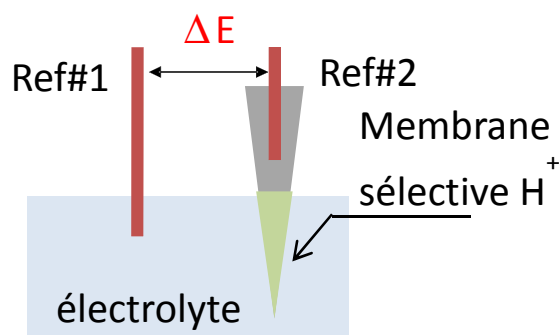
Figure II- 7 : Représentation schématique du principe de mesure de la microélectrode de pH.
