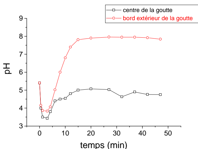
Figure II- 6- Variation du pH de surface dans une goutte d'eau de 5mm de diamètre sur un alliage Al-Cu (2011). Mesure avec une sonde pH type W/WO 3 (250 μm) [9].
