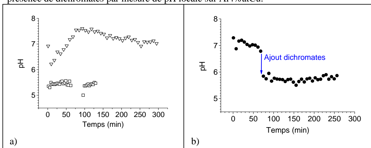
Figure III- 45 : Evolution du pH à la surface d'une solution solide Al4%atCu-Décapage au préalable 15 s dans NaOH 0.5mM ; (a) (∇) NaCl 0,1M ; (□) NaCl 0,1M + K_2Cr_2O_7 10^{-4}M ; (b) (●) NaCl 0.1M puis après 70 min ajout de 0.2 ml de K_2Cr_2O_7 10^{-3}M + NaCl 0.1M (concentration globale de 3 \cdot 10^{-4}M ).
