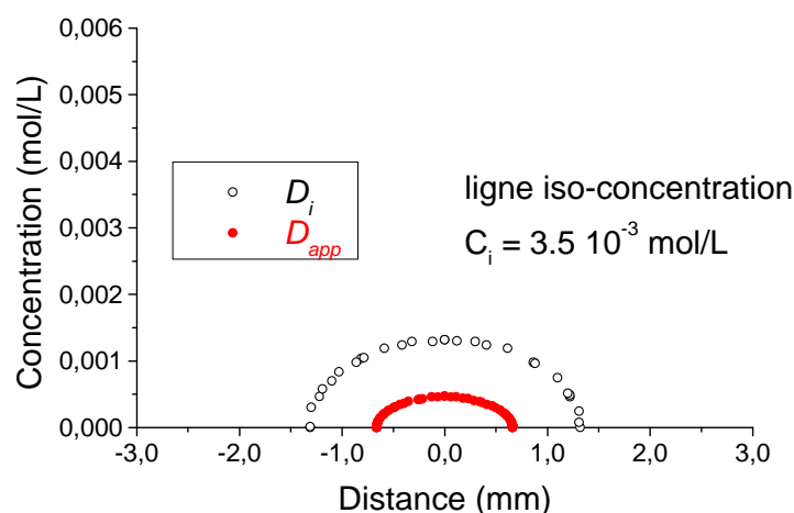
Figure V- 9: Portée du couplage chimique selon que le transport est sous contrôle diffusional pur (○) ou dans un régime de diffusion convective (●);(Tableau V-1 ; géométrie b)
