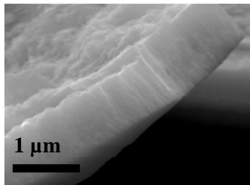
Figure II- 4 : Observation sur la tranche d'un dépôt PVD (écaille) d'épaisseur 1μm.
