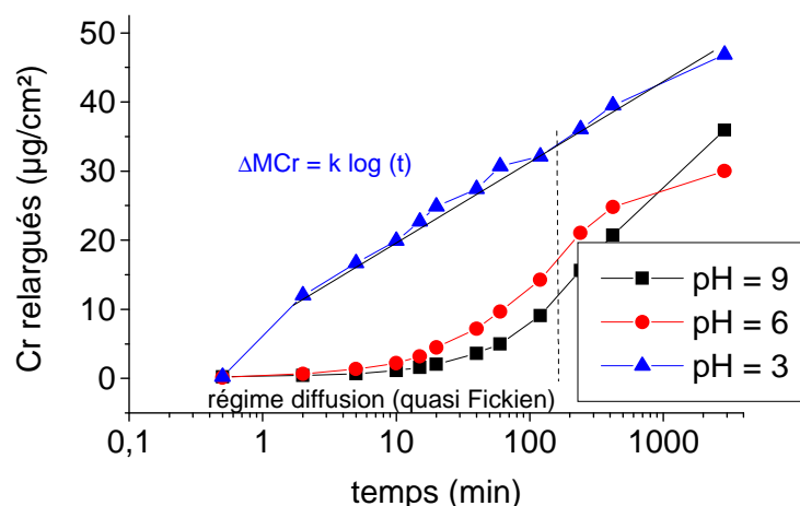
Figure IV- 6 : Représentation en échelle logarithmique de la Figure IV- 5 représentant l'évolution de la concentration en dichromates pour différents pH soit Q_{diss} = k \log(t) .
