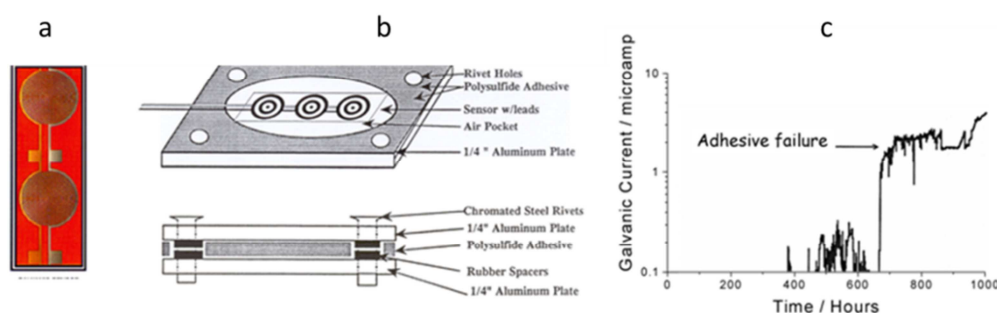
Figure I- 57 : Capteur d'alerte de risque de délamination ; a) Capteur environnemental de type capteur de type couple galvanique (par exemple or et fer, or et zinc, ... ) ; b) Schéma d'insertion du capteur dans une zone de recouvrement de tôles ; c) Réponse du capteur dans un test de brouillard salin [74].
