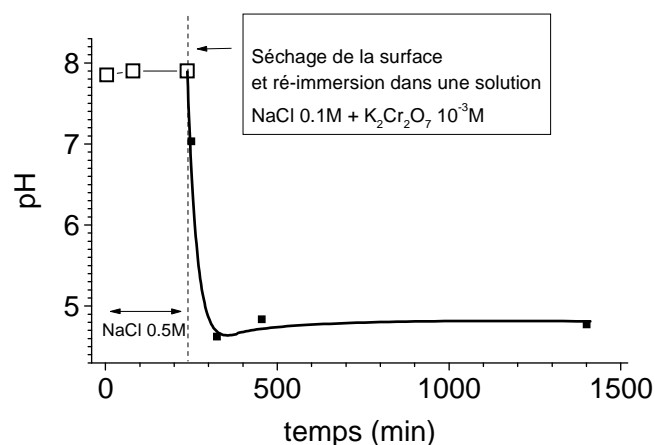
Figure III- 10 : Variation du pH de surface (distance sonde-surface = 150 \mu m) au centre de l'échantillon immergé successivement dans une solution chlorurée sans puis avec dichromates. La concentration en dichromates de la seconde solution chlorurée est de 10^{-3}M et son pH = 4.75.
