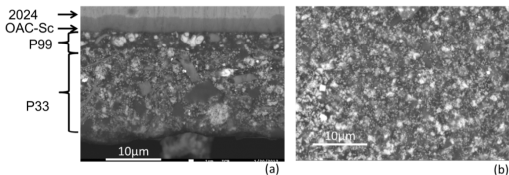
Figure IV- 1 : Observation MEB ; a) sur la coupe travers court (tranche) d'un alliage 2024 revêtu d'une couche OAC-Sc et de deux peintures chromatisées (Ech #3), b) sur la face externe d'un alliage 2024 revêtu d'une couche d'OAC-Sc et d'une peinture contenant des dichromates (Ech #5).
