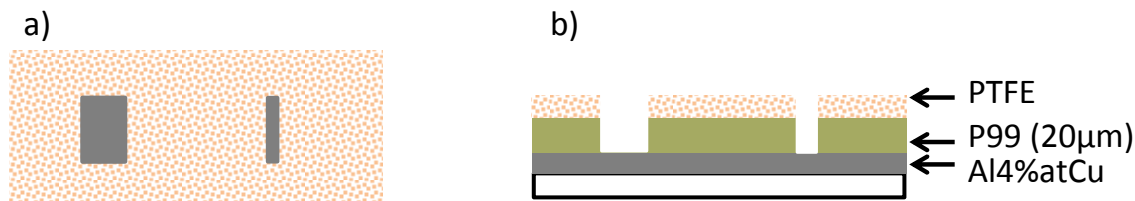
Figure II- 22 : Représentation schématique de l'échantillon après l'étape d'application de P99 et la mise en place des masque de téflon ; a) vue du dessus ; b) vue de côté.
