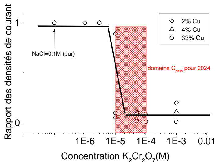
Figure III- 59 : Définition du domaine d'efficacité des dichromates pour les différentes solutions solides Al-Cu (courant de réduction mesuré à E=-1.2 V / Ag-AgCl ). Leur domaine de passivation est voisin de celui obtenu pour l'alliage 2024 (Figure III- 20).
