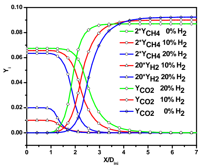
Figure 7.30 Evolution des espèces sur l'axe de symétrie
