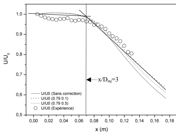
Figure 7.6 Vitesse axiale
