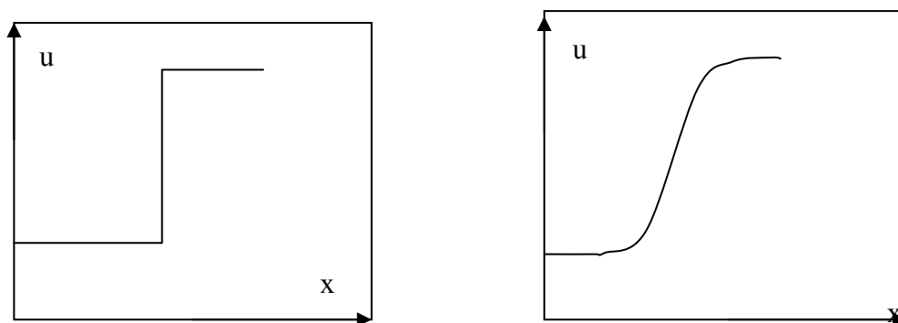
Figure 6.3 Fausse diffusion induite par le schéma amont du premier ordre
