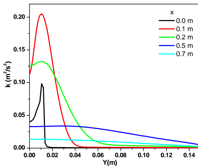
Figure 7.11 Distribution radiale de l'énergie de turbulence pour l'écoulement non réactif à différentes positions x
