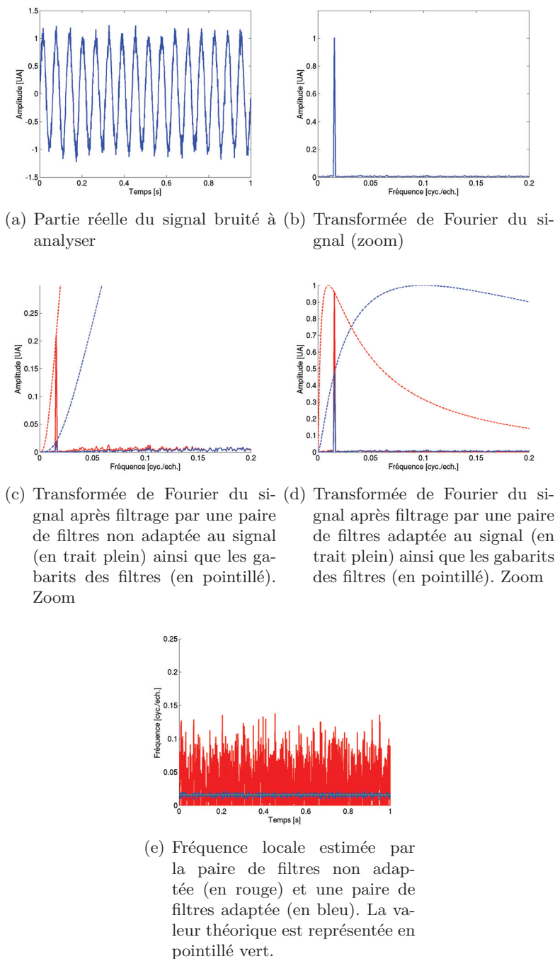
FIG. 6.2: Exemple d'application de la méthode proposée par H. Knutsson et al. avec deux paires de filtres l'une adaptée et l'autre mal adaptée sur un signal bruité. Le signal à analyser a une fréquence de f = 0,015 \text{ cyc./ech.} sur toute la durée de l'acquisition et un SNR de 20 \text{ dB} . Les deux filtres R_{\xi_0} et R_{\xi_1} ont respectivement pour fréquences centrales : 0,1 \text{ cyc./ech.} et 0,3 \text{ cyc./ech.} (soit C_B = 0,455 ) pour la paire de filtre mal adaptée et 0,01 \text{ cyc./ech.} et 0,1 \text{ cyc./ech.} (soit C_B = 0,217 ) pour les deux filtres bien choisis. Le zoom sur le graphique (c) met en valeur le fait que la puissance de la fréquence utile filtrée par le filtre représenté par la courbe bleue est du même ordre de grandeur que le bruit, impliquant une mauvaise estimation de la fréquence utile. La valeur moyenne de la valeur absolue de l'erreur est MAE = 0,0019 \text{ cyc./ech.} pour la paire de filtres bien choisie et MAE = 0,058 \text{ cyc./ech.} pour la paire de filtres mal adaptée.
