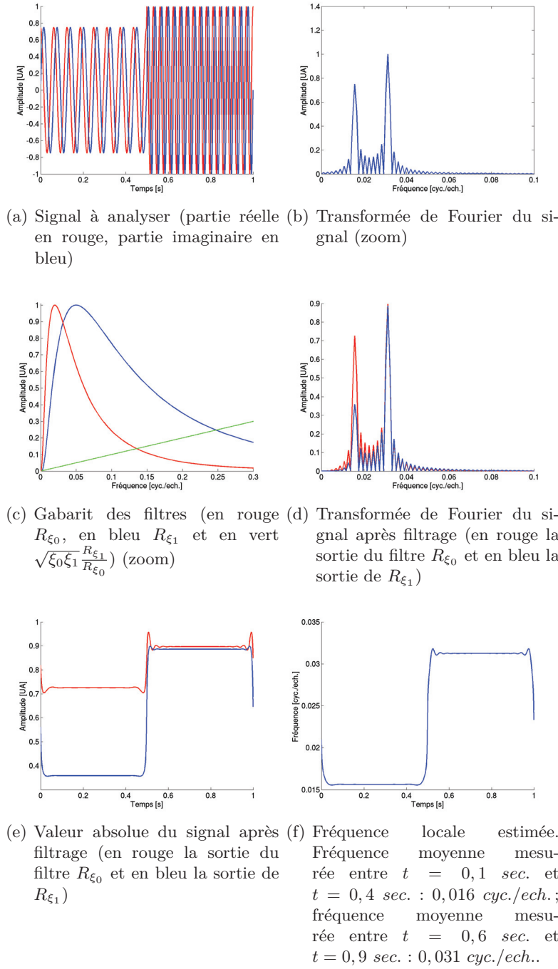
FIG. 6.1: Exemple d'application de la méthode proposée par H. Knutsson et al. avec une seule paire de filtres. Le signal à analyser a une fréquence de f = 0,016 \text{ cyc./ech.} avec une amplitude de 0,75 pour t \in [0, 0,5[ \text{ sec.} et une fréquence de f = 0,031 \text{ cyc./ech.} avec une amplitude de 1 pour t \in [0,5, 1[ \text{ sec.} . Les fréquences sont données en fréquences normalisées (entre 0 et 1 ). Les deux filtres R_{\xi_0} et R_{\xi_1} ont respectivement une fréquence centrale de 0,02 \text{ cyc./ech.} et 0,05 \text{ cyc./ech.} (soit C_B = 0,546 ). Les amplitudes sont données en unité arbitraire ( UA ).
