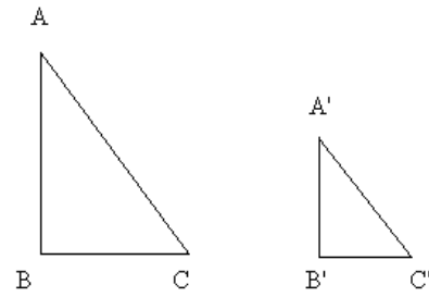
Figure 4 : Deux triangles semblables
