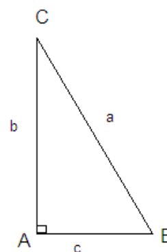
Figure 1 : Triangle rectangle à
