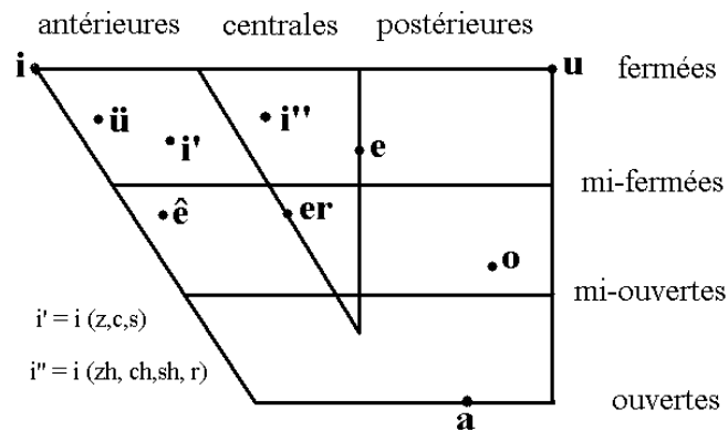
Schéma 9 : Schéma articulatoire des voyelles chinoises
