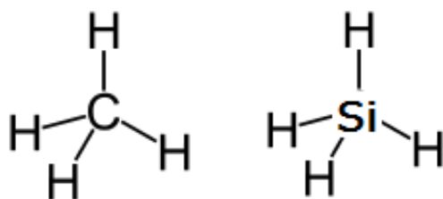
Figure 3 : Molécules de méthane et de silane
